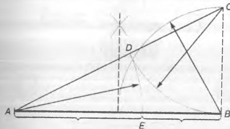
Построение золотого сечения
