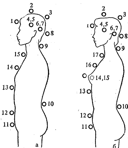
Рис. 1.17. Чакры мужчины (а) и женщины (б).
