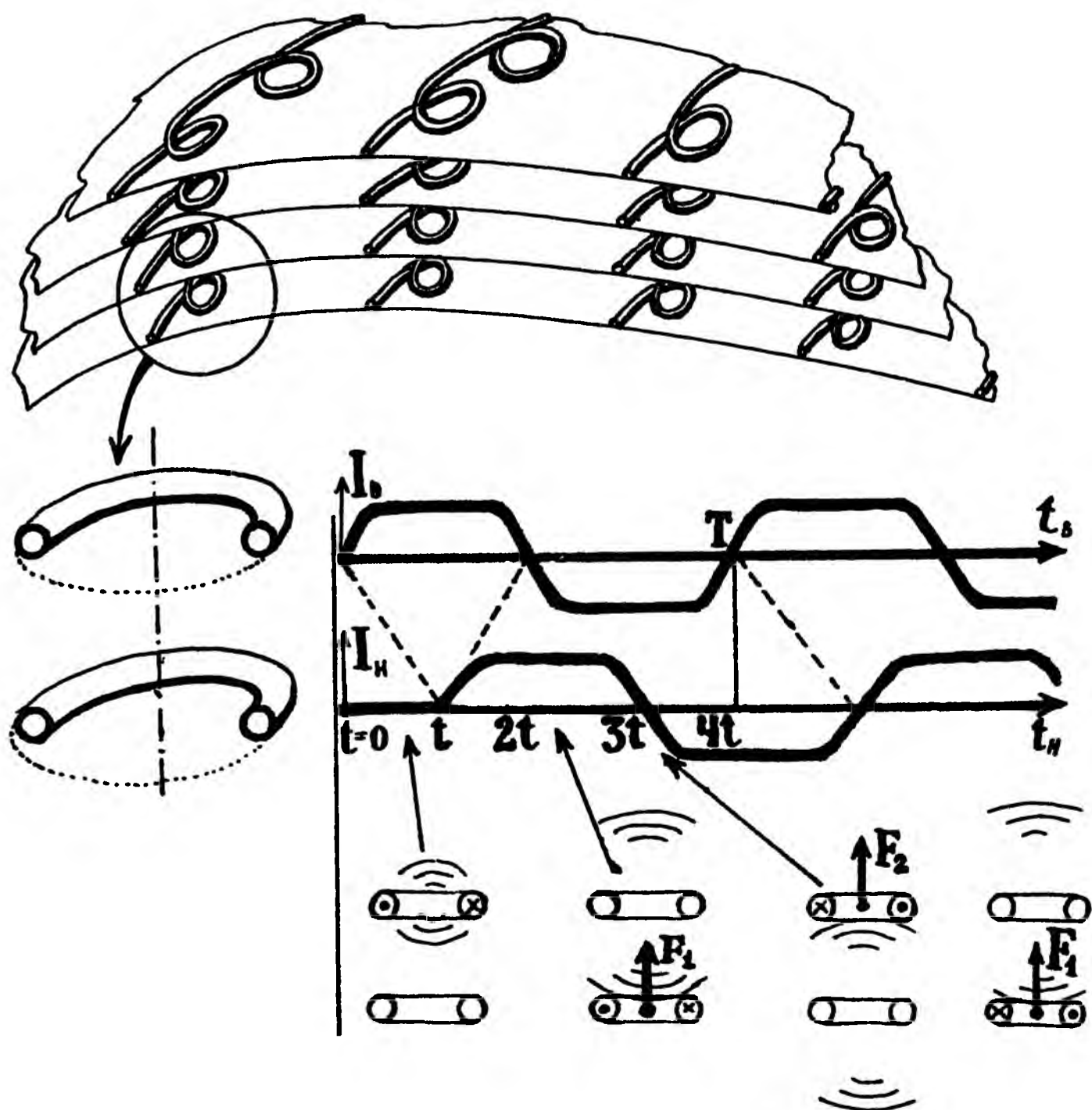
Рис. 19. Электромагнитная рабочая поверхность (ЭРП)
