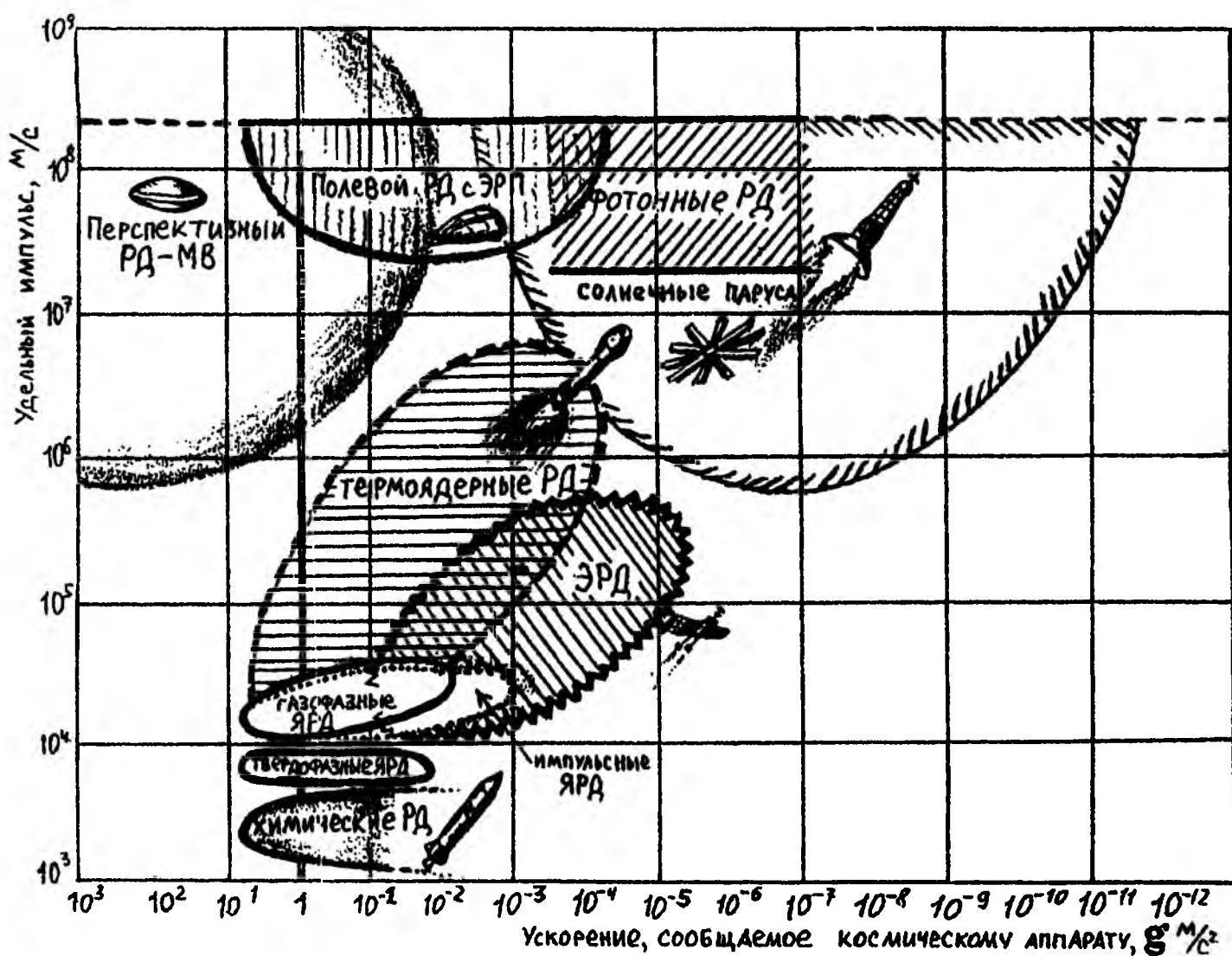
Рис. 48. Сравнение тактико-технических характеристик двигателей на основе машины времени и других перспективных проектов
