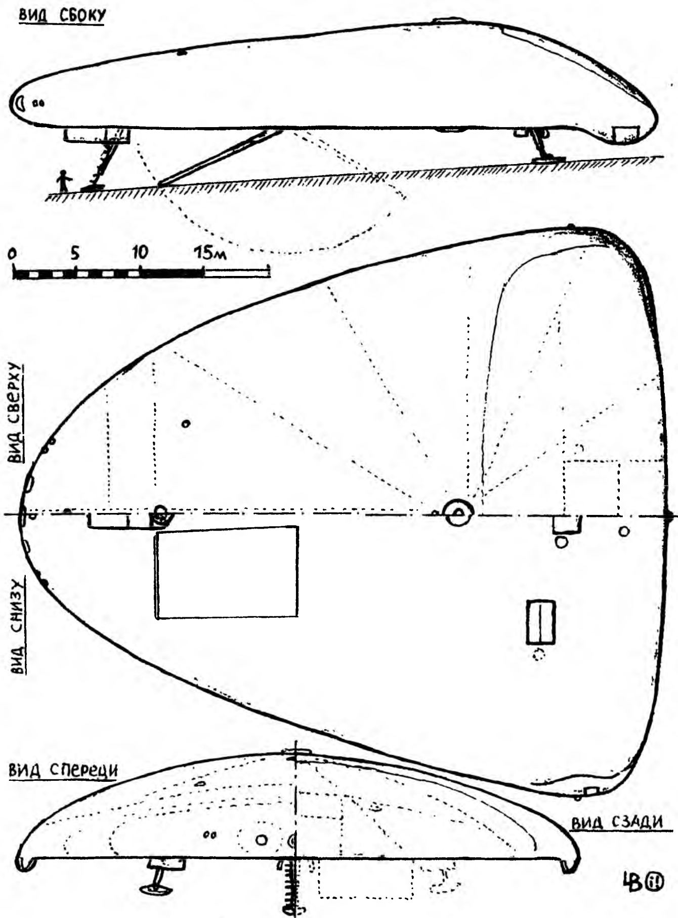
Рис. 28. Схема летательного аппарата «Ирма-7» (проект 1992 года)
