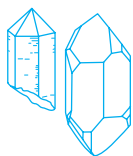
SiO 2
