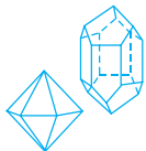
SiO 2
