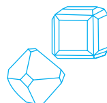
Cu
