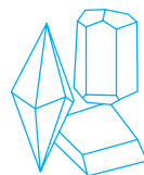
CaCO 3
