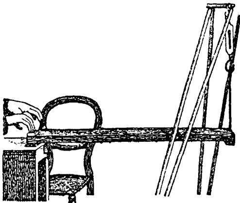
Рис. 62. Прибор для измерения изменений веса
