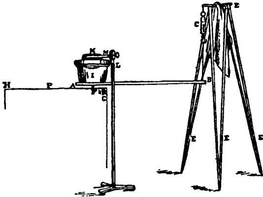
Рис. 64. Другой прибор Крукса для взвешивания
