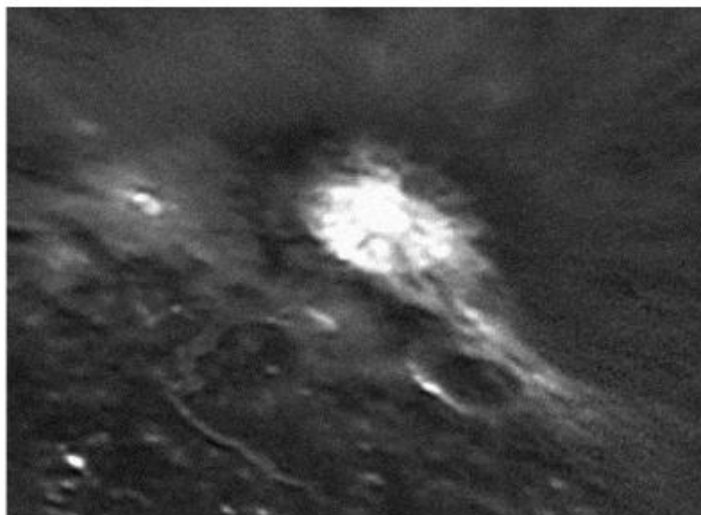
Голубой свет на дне кратера Аристарх 17 декабря 2005 г. Фото Mike's Astroimagery UK
