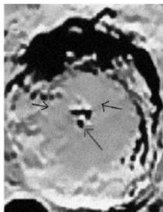
Непонятные сооружения прямоугольной формы на дне лунного кратера. www.rense.com
