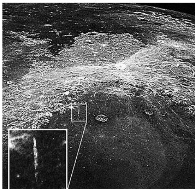
Башня высотой 20 миль, как бы вырастающая из Моря Кризисов. Фото, продемонстрированное Ричардом Хогландом. Снимок сделан в рамках программы «Аполлон-16»
