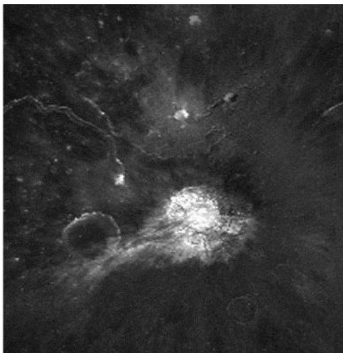
Голубой свет на дне кратера Аристарх в 1994 г. Фото с космического корабля «Clementine», НАСА. Обратите внимание на расположенную на обоих фото в центре кратера куполовидную структуру, из которой изливается свет и освещает прилегающие участки кратера, а также на несколько небольших локальных источников света на дне кратера
