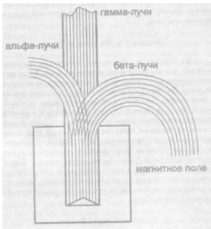
Рис.2. Разделение излучения радия в магнитном поле.
