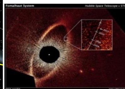
Рис. П7-13а Fomalhaut и Fomalhaut B
