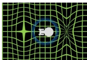
Рис. П7-16 «Пузырь Алькубьерре»
