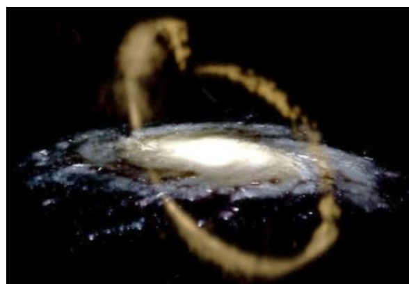
Рис. П7-12а Истекающий поток из карликовой галактики в Большом Псе
