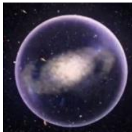
Галактика
