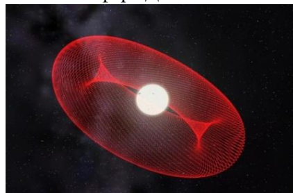
Рис. П7-17в Пузырь Дайсона
