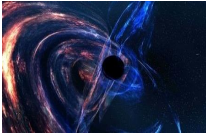
Чёрная дыра
