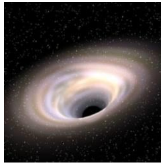
Рис. П7-25а Черная дыра в системе Лебедь X-1 и V404 Cygn (илл. NASA /CXC/ M. Weiss)
