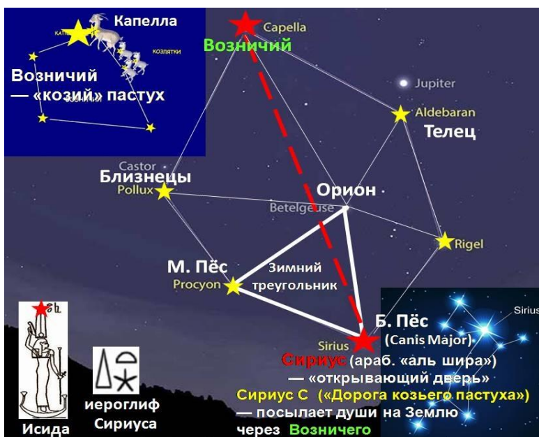
Рис. П7-17а Сириус – Возничий 71
