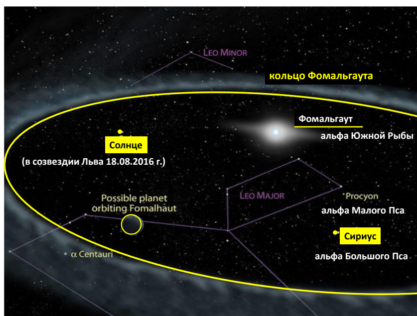
Рис. П7-13 Кольцо Фомальгаута
