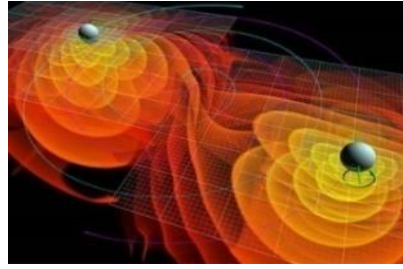
Две чёрные дыры
