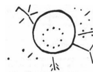
Сириус В (зерно «По») звезда «Дигитария» 22
