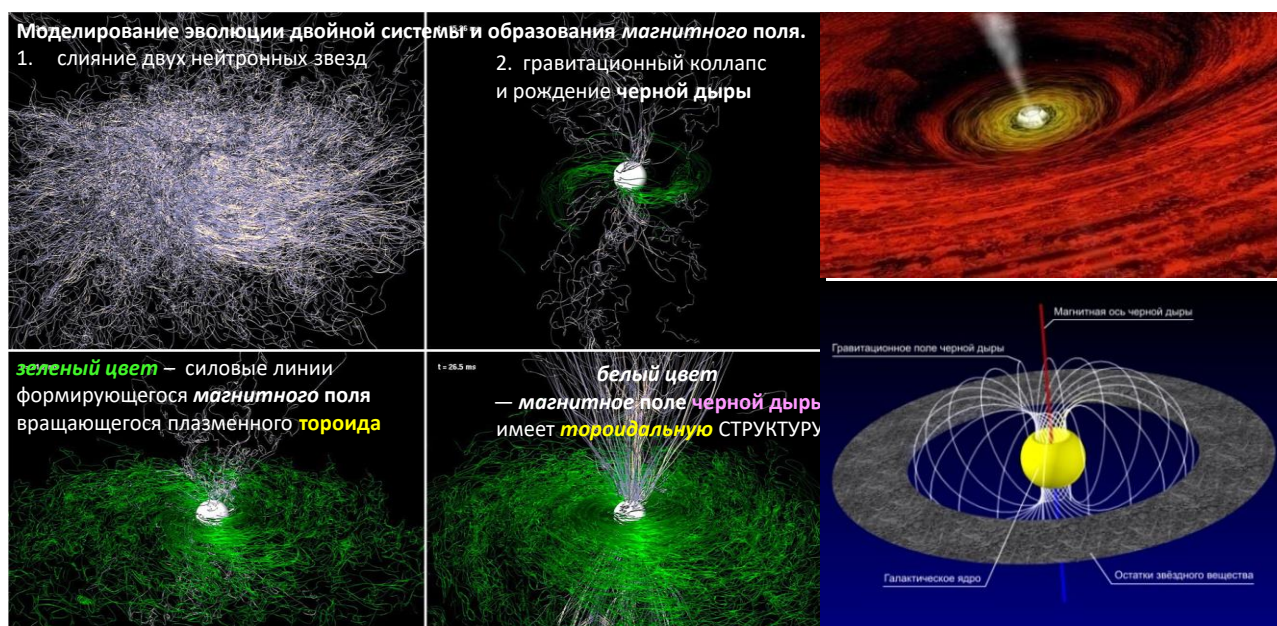
Рис. П7-5а Магнитное поле чёрной дыры
