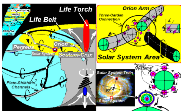
Рис. 23 Тор Галактики «Млечный Путь», Солнце в рукаве Ориона
