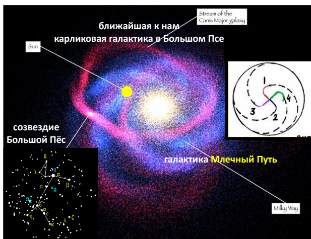
Рис. П7-12 Карликовой галактики в Большом Псе
