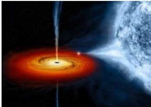
Рис. П7-25а Черная дыра в системе Лебедь X-1 и V404 Cygn (илл. NASA /CXC/ M. Weiss)
