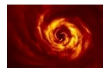
Рис. П7-13в Possible planet*
