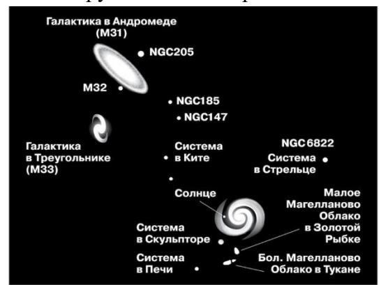
Рис. П7-3а Местная группа галактик 2
