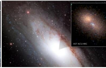
Ядро Андромеды
