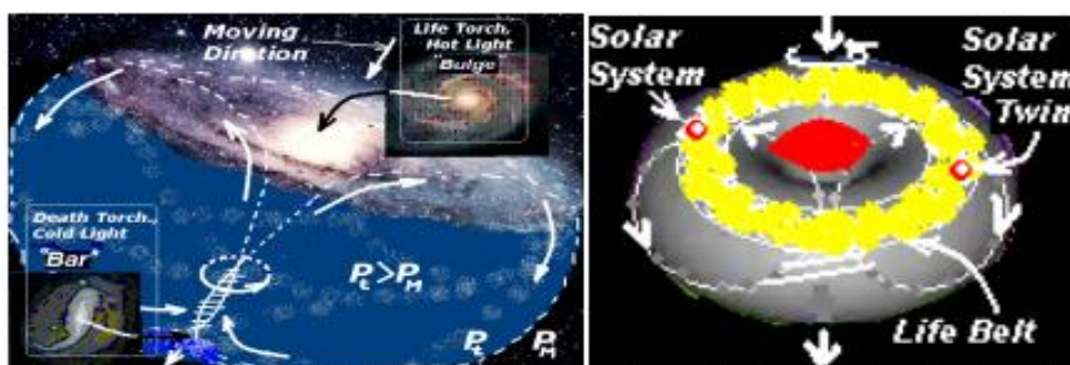
Рис. 9 Действующая галактика «Туманность Андромеды (слева) и местоположение «Пояса Жизни» в любой действующей галактике (справа)
