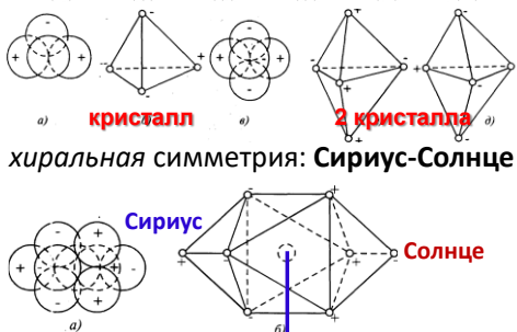
Рис. П7-8а Ячейка Анубиса
