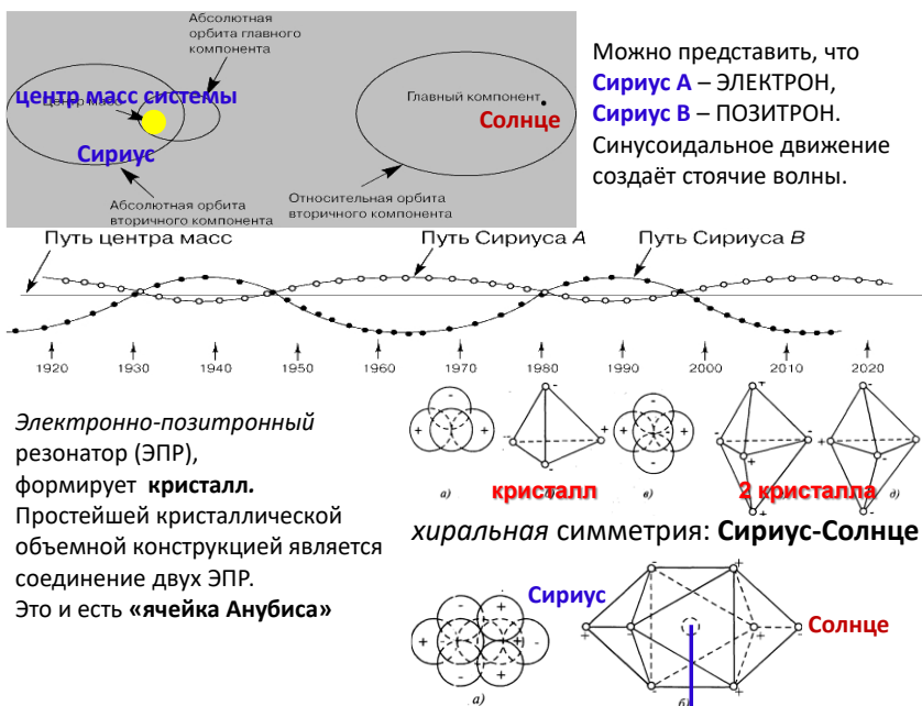
Рис. П7-8а Ячейка Анубиса
