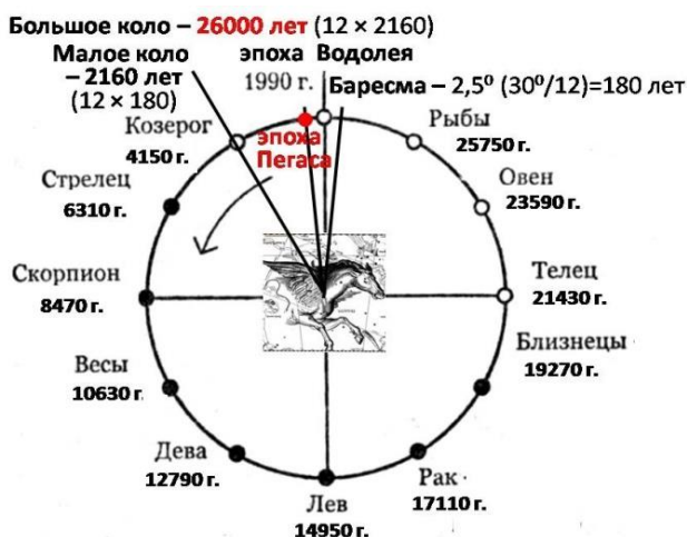
Рис. П7-14 Большое коло
