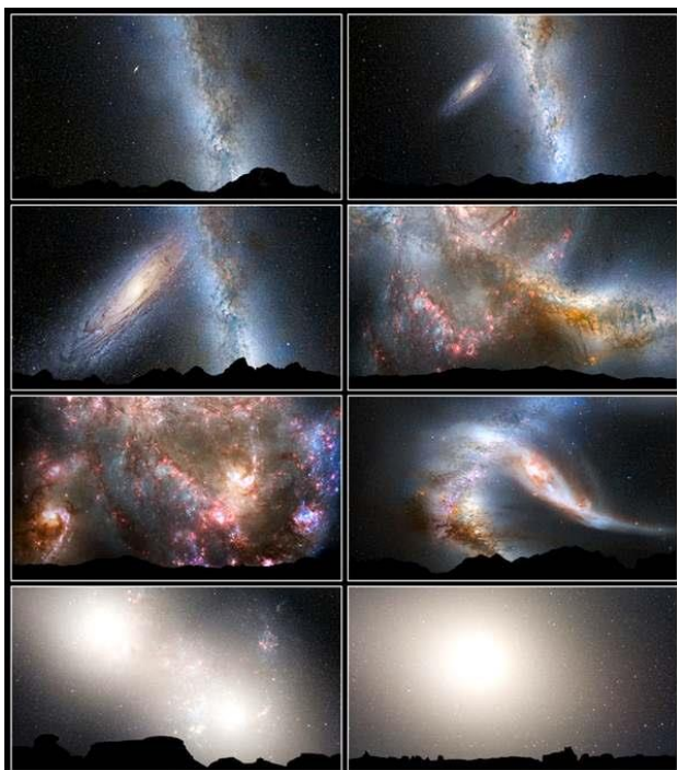
Рис. П7-1 Столкновение галактик Млечный Путь и Андромеды (M31)
