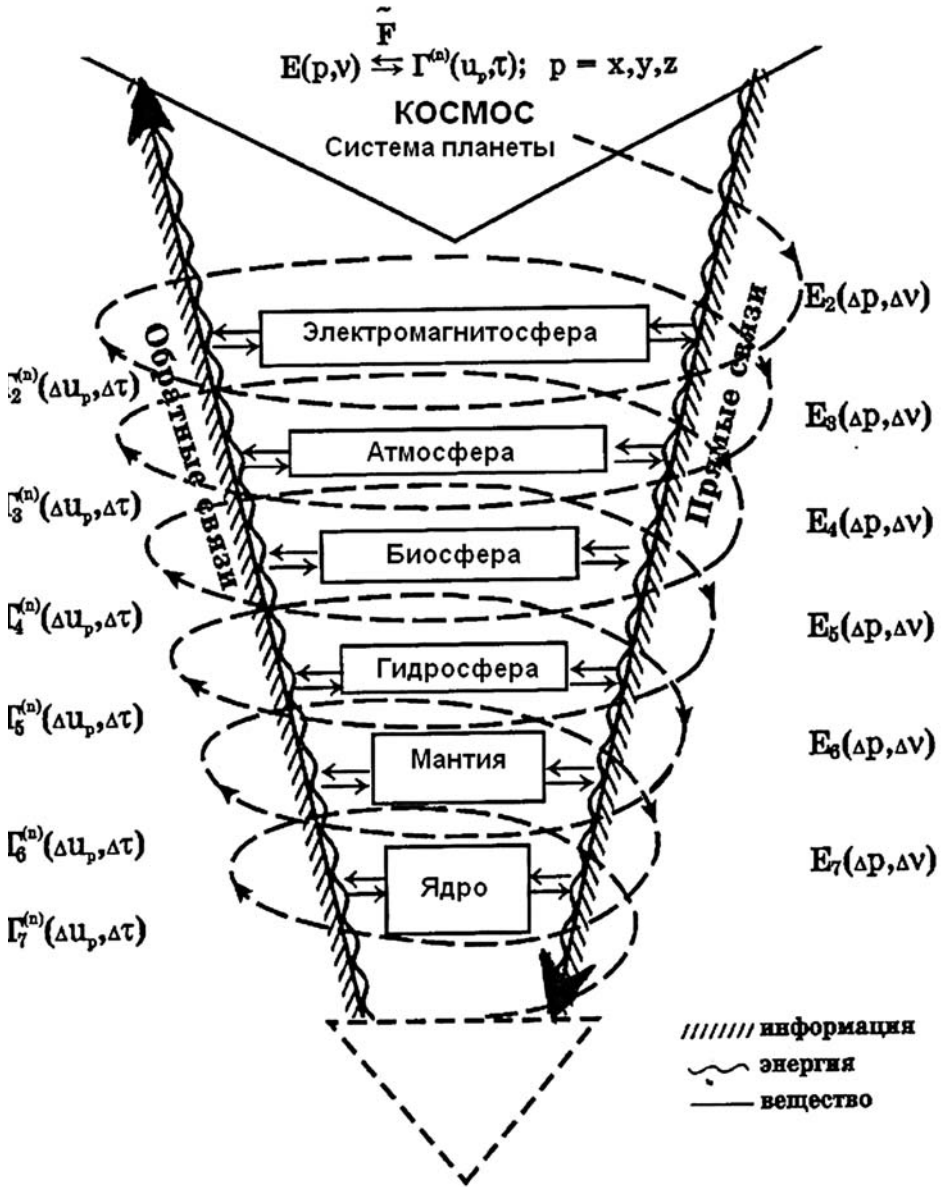
Рис. 2. Геосферная Иерархическая Цепь
