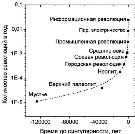
Рис. 1. Наглядное представление сингулярности эволюции и существования режима с обострением: точки — несколько последних фазовых переходов; ось ординат — количество фазовых переходов в год; ось абсцисс — абсолютное время фазового перехода, отсчитанное от точки сингулярности
