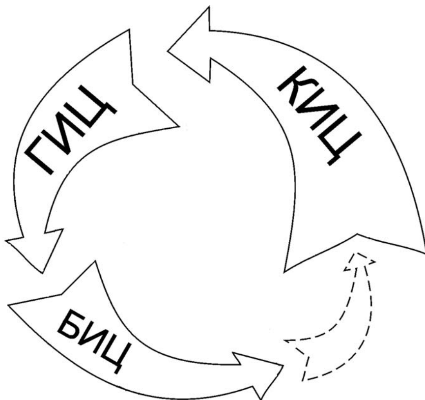
Рис. 4. Единая всемирная цепь взаимодействий
