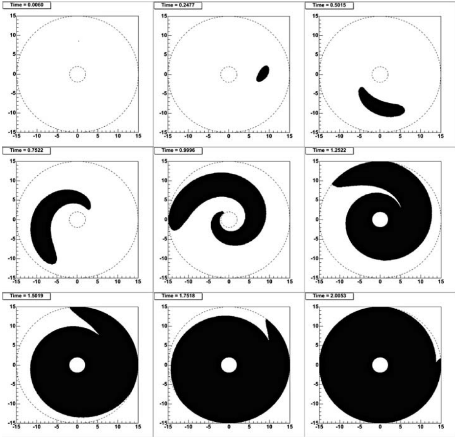
Рис. 4. Численная модель распространения волны панспермии в Галактике: время в галактических годах; оси координат – расстояние в килопарсеках; расчет проведен для звезды – источника инфекции, находящейся на таком же расстоянии от центра Галактики, как Солнце
