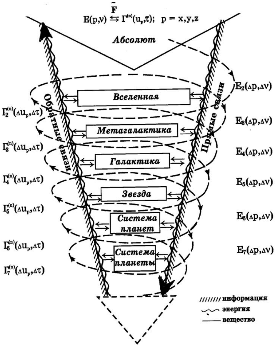
Рис. 1. Космическая Иерархическая Цепь. Описание приведенных на схеме обозначений дано в приложении
