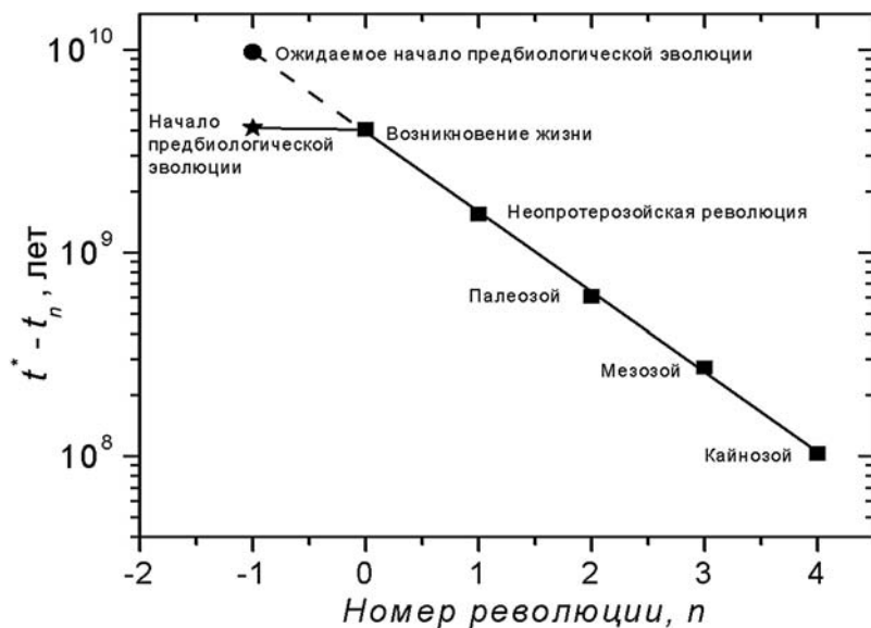
Рис. 3. Аномалия «ключки» в общей масштабнo-инвариантной эволюции биосферы
