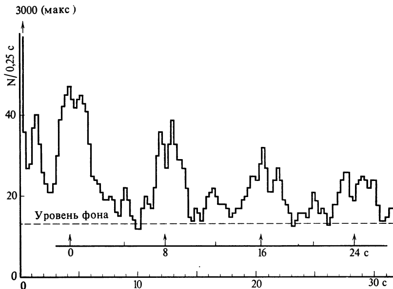
Рис. 48. Мощный всплеск и последующее пульсирующее затухание рентгеновского излучения, зарегистрированное станцией «Венера-12» 5.III 1979 г.
