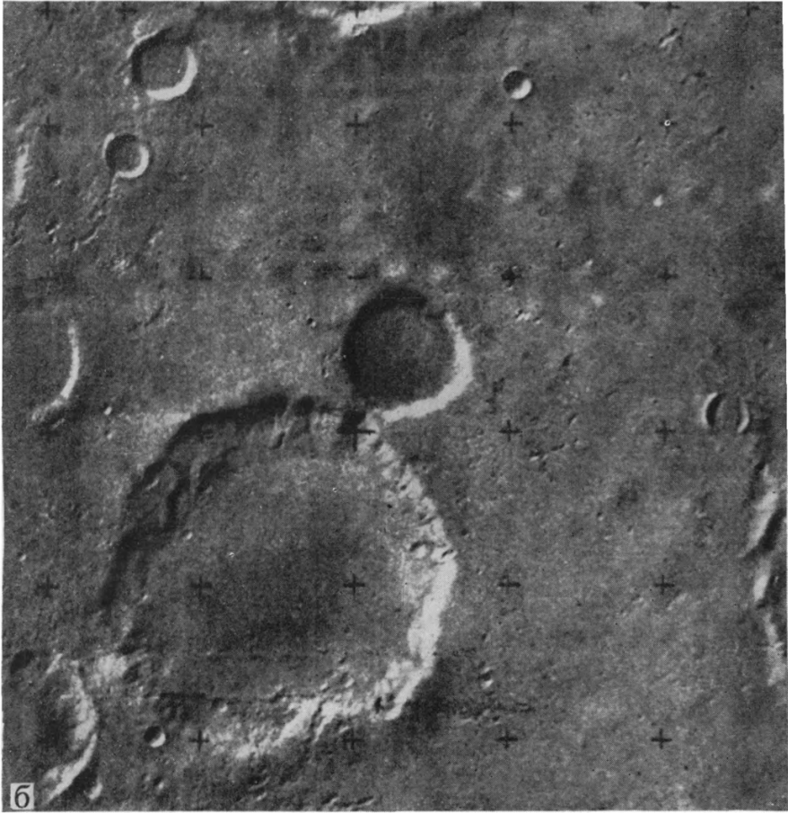
к западу меандрирующая долина Нергал. В центре снимка кратеры Бонд и Хейл; 6 — снимок участка кратерированной равнины к северо-востоку от кратера Бонд (координаты центра 32^{\circ} ю. ш., 33^{\circ} з. д.), для которой характерны неглубокие линейные депрессии на поверхности. Наибольший кратер имеет диаметр \sim 35 км, у него плоское дно
