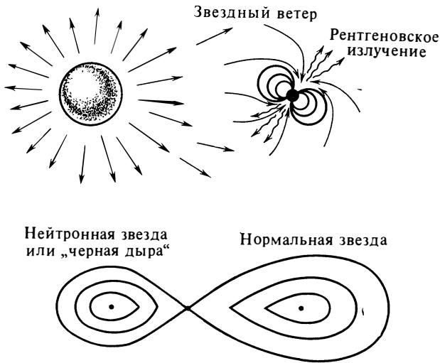
Фиг. 47. Механизм генерации рентгеновского излучения в тесной двойной системе (модель)
