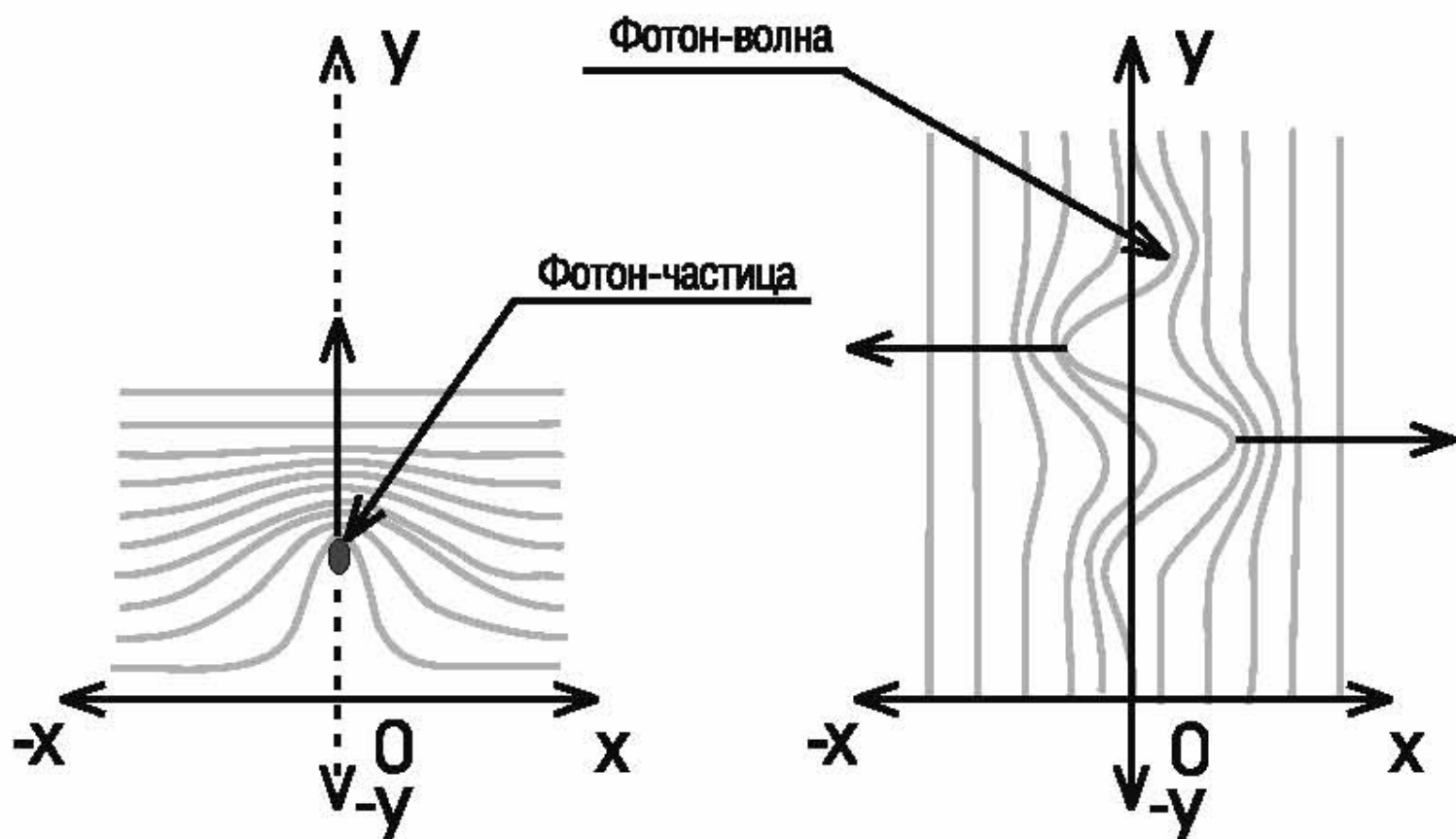
Рис. 14. Деформация гравитационно-спинового пространства фотоном:
