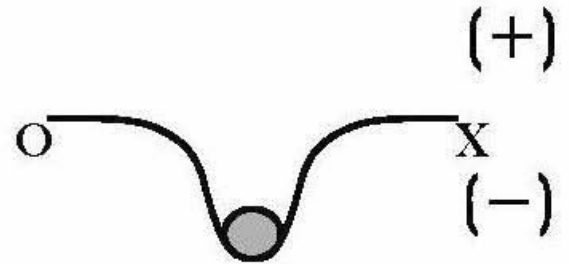
Рис. 2. Гравитационная потенциальная «яма» в (+) подпространстве, как прогиб пространственной мембраны образованный телом положительной массы (серый кружок).
