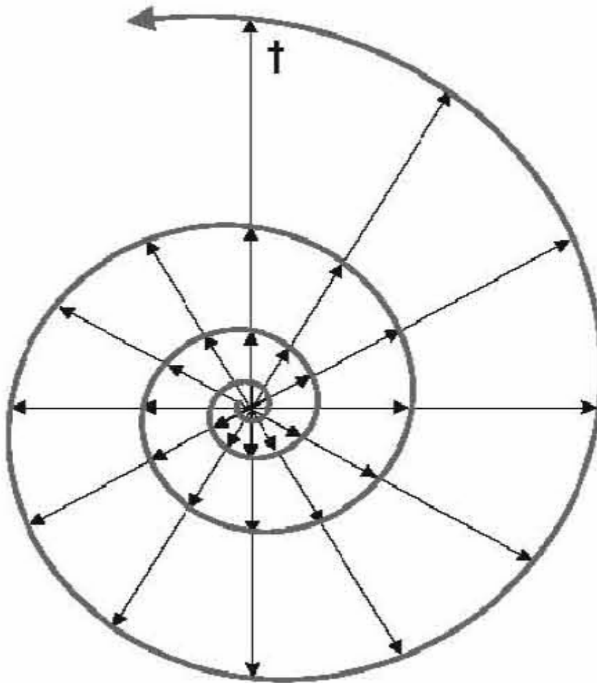
Рис. 19 Эволюция самоорганизованных тел и систем микро, макро и мегамира, как движения стрелы времени по расходящейся спирали в "четырёхликом" пространстве-времени.
