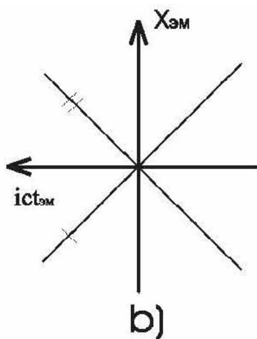
б) Результат поворота пространства Минковского на 90^\circ приводит к трансформации гравитационно-спинового пространства времени в электромагнитное, с координатами X_{\text{эм}} , i\text{ct}_{\text{эм}} .
