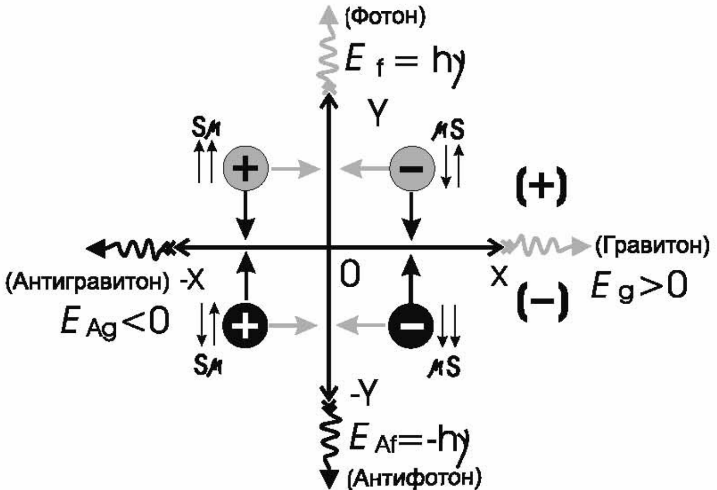
Рис. 11. Показана схема аннигиляции четырёх видов частиц (электрона) в (+) и (-) подпространствах. Стрелками показано направление спина и магнитного момента частиц и античастиц. Встречными стрелками показано направление аннигиляции частиц, различа-
