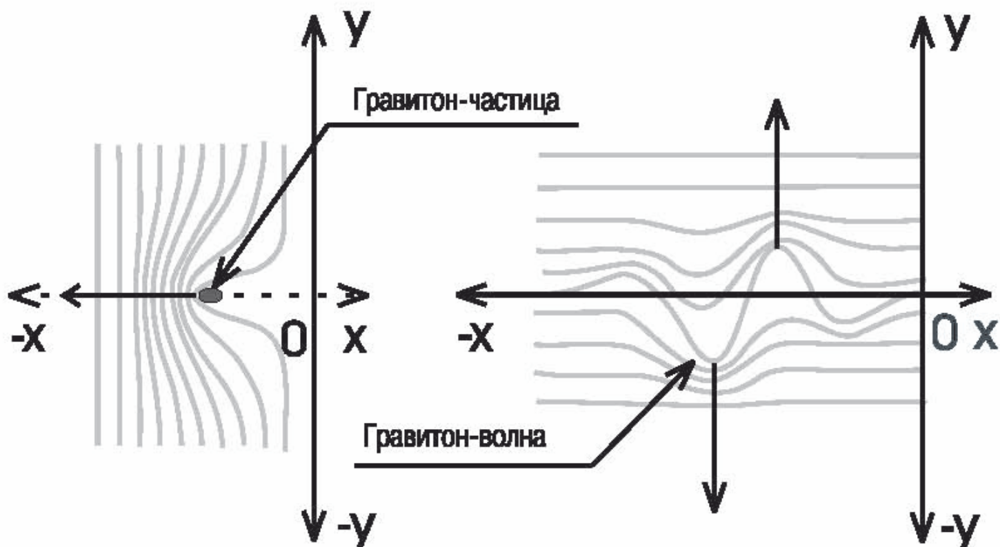
Рис. 15. Деформация электромагнитного пространства гравитоном:
