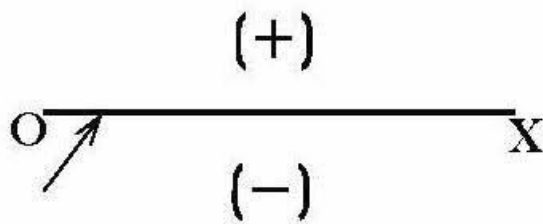
Рис. 1. Стрелкой показано сечение пространственной мембраны, разделяющей пространство на два подпространства (+) и (-).
