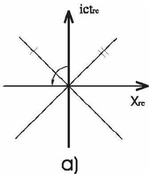
Рис. 17 а) Показан поворот пространства Минковского против часовой стрелки. Штрихами обозначены мировые линии. X_{\text{гс}} и i\text{ct}_{\text{гс}} пространственная и временная координаты гравитационно-спинового пространства.
