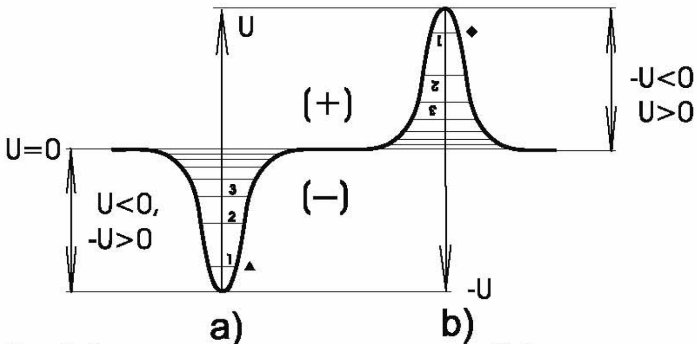
Рис. 9. Упрощенная картина распределения потенциальной энергии в двух зеркальных, симметричных, подпространствах: а) для обычного электрона в атоме (+) подпространства; б) для антипозитрона в антиатоме (-) под-
