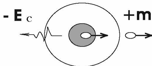
Рис. 8 Вынос положительного вещества и отрицательной свободной энергии из потенциальной «ямы» (-) подпространства.
