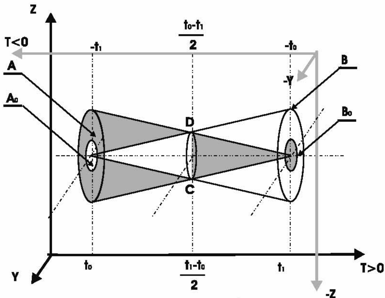
Рис. 21. Показано два зеркально симметричных подпространства (представленных в двумерном виде с координатами Y и Z ), в которых происходит эволюция "положительных" и "негативных" компонент самоорганизованной системы. Её развитие идёт в двух противоположных направлениях времени (показано в виде белого и серого конусов рассеяния). Тело A_0 (выделено малым белым
