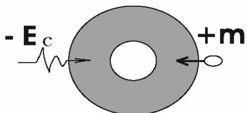
Рис. 5 Аккреция положительного вещества +m и отрицательной свободной энергии (показана извилистой стрелкой) в гравитационную потенциальную «яму» (+) подпространства.
