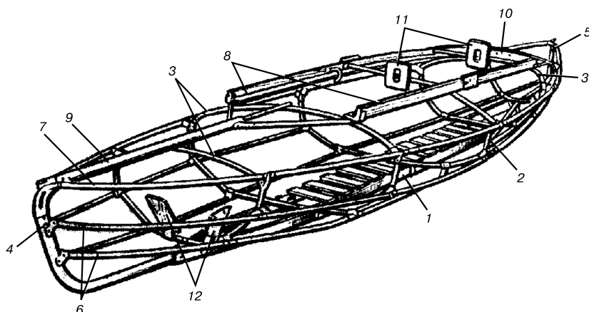
Рис. 4.3. Каркас байдарки:
