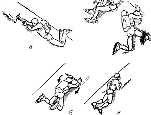
Рис. 22. Самозадержание на льду: a – клювом ледоруба; б – на пористом льду клювом и штычком; в – классический приём
