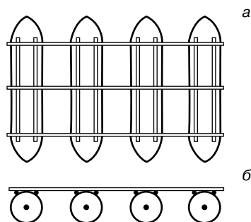
Рис. 4.8. Плот на поперечных гондолах: а – вид сверху; б – вид сбоку
