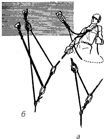
Рис. 18. Система полиспаста: a – варианты одинарного полиспаста; б – двойной полиспаст
