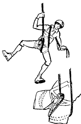
Рис. 29. Спуск на верёвке: а – с применением восьмёрки; б – с применением шайбы Штихта
