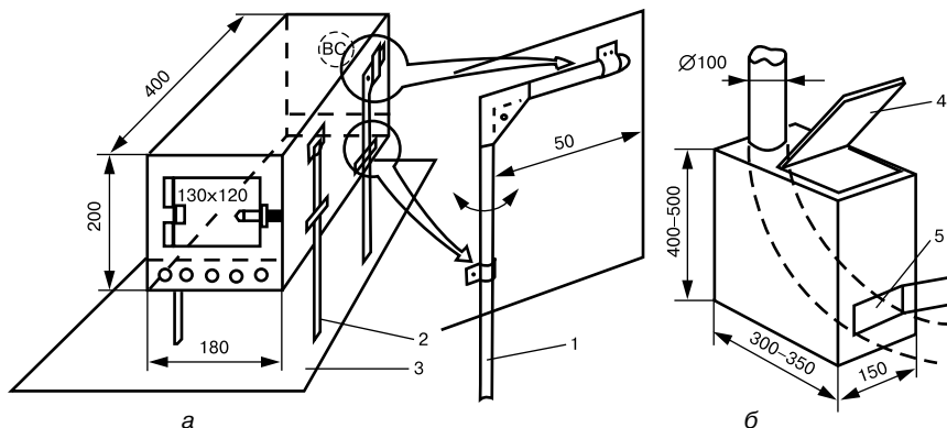
Рис. 6.8. Смонтированные печи:
