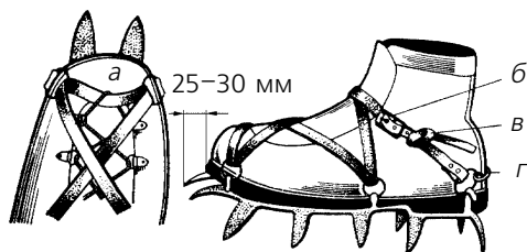
Рис. 1. Крепление кошек к ботинкам: а – фиксация носкового ремня; б – пряжка с наружной стороны ботинка; в – фиксирующий узел; г – пяточная скоба
