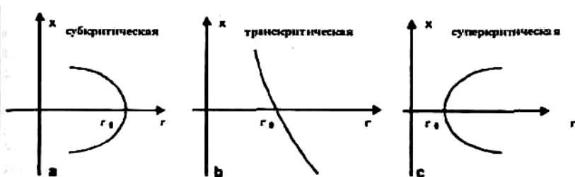
Рис. 3.18. Простые точки бифуркации.
