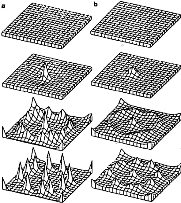
Рис. 8.14. Двумерная модель морфогенеза: а) концентрация активаторов; б) концентрация ингибитора.
