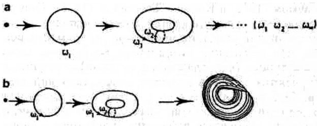
Рис. 6.1.(a) Переход к хаосу по Ландау. (b) Переход к хаосу по Рюэлю-Такенсу—Ньюхаусу.
