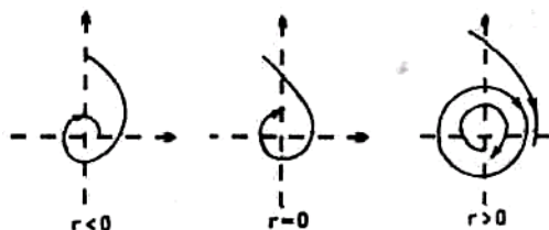
Рис. 3.13 Бифуркация Хопфа.
