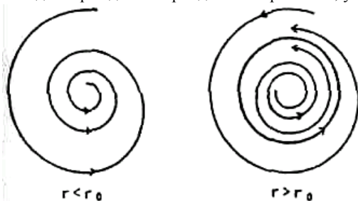
Рис. 5.3. Фазовый портрет системы (5.2.9) при r_0 = 0 .
