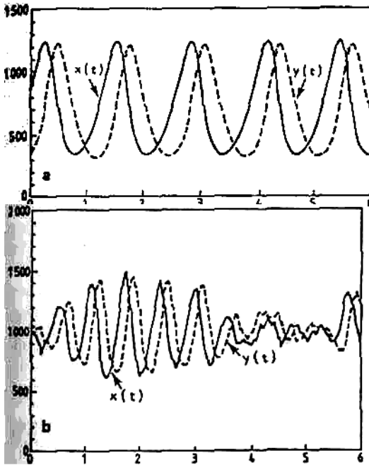
Рис. 7.2. Временные зависимости в системе (а) детерминированных уравнений, (б) стохастических уравнений.
