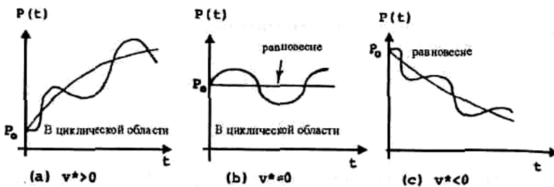
Рис. 5.8. Осцилляции цен.
