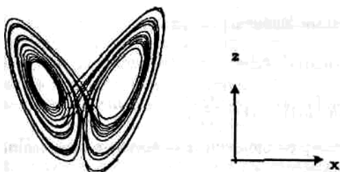
Рис. 6.9. Хаотическая динамика города.
