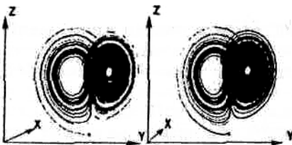
Рис. 6.8. Аттрактор Лоренца.
