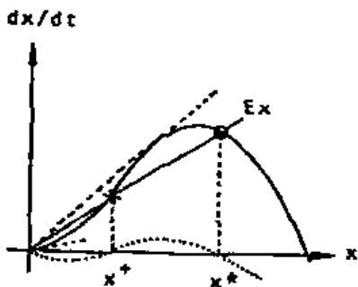
Рис. 4.7. Случай некритического воспроизводства.
