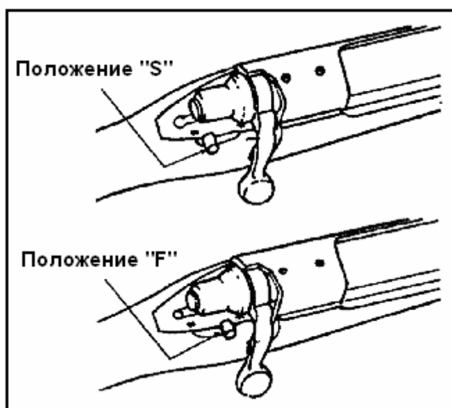
Рис. 2-3. Предохранитель.
