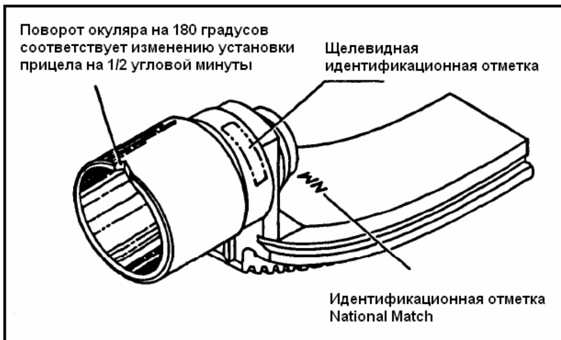
Рис. В-3. Прицельное приспособление National Match.
