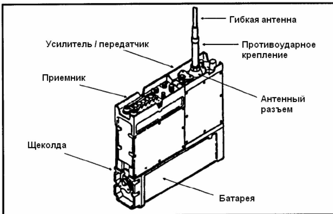
Рис. 2-35. Приемопередатчик AN/PRC-104A.
