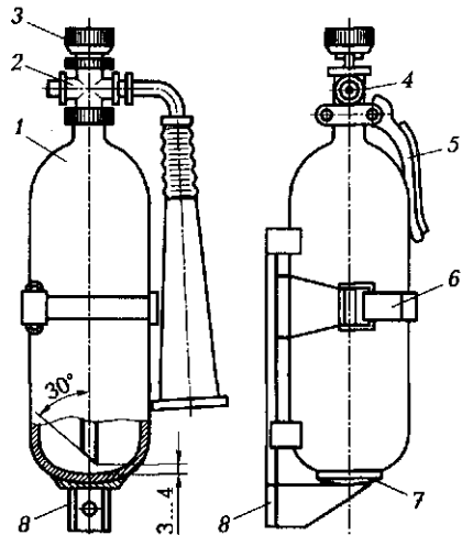
Рис. 2.3. Углекислотный огнетушитель ОУ-2:
