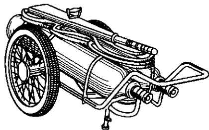
Рис. 2.4. Передвижной углекислотный огнетушитель УП-2М
