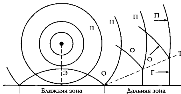
Рис. 1.3. Образование ударной волны при воздушном взрыве:
