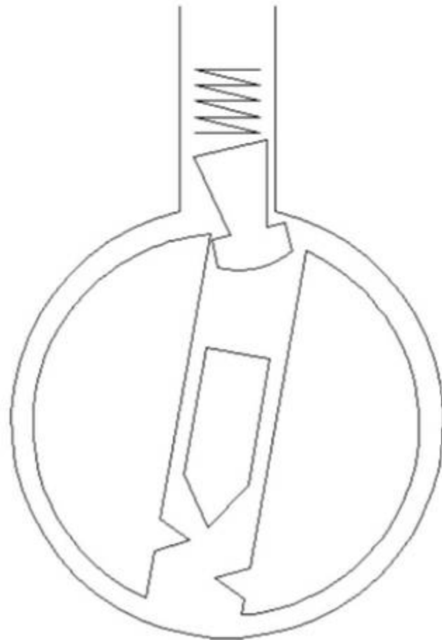
Рис. 9.7 Грибовидные, катушковидные и пильчатые направляющие штифты
