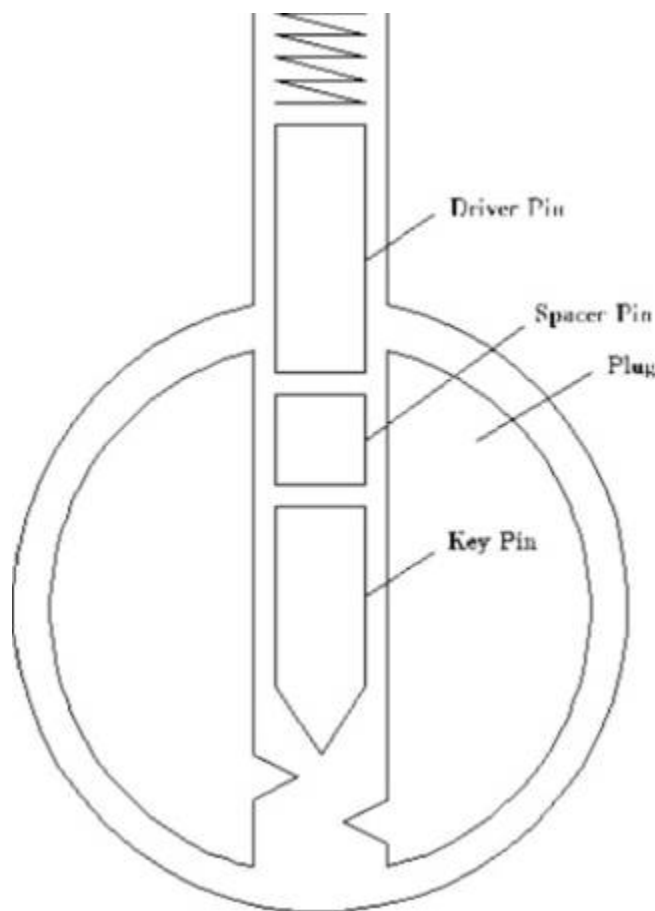
Рис. 9.8 Промежуточные штифты для мастер-ключей
