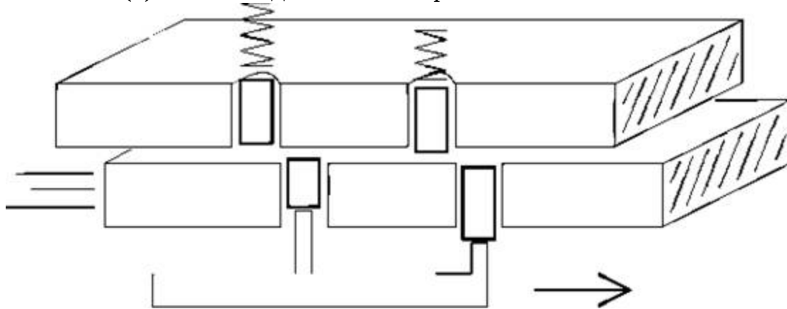
Рис. 3.2 (а). Ключ поднимает штифты
