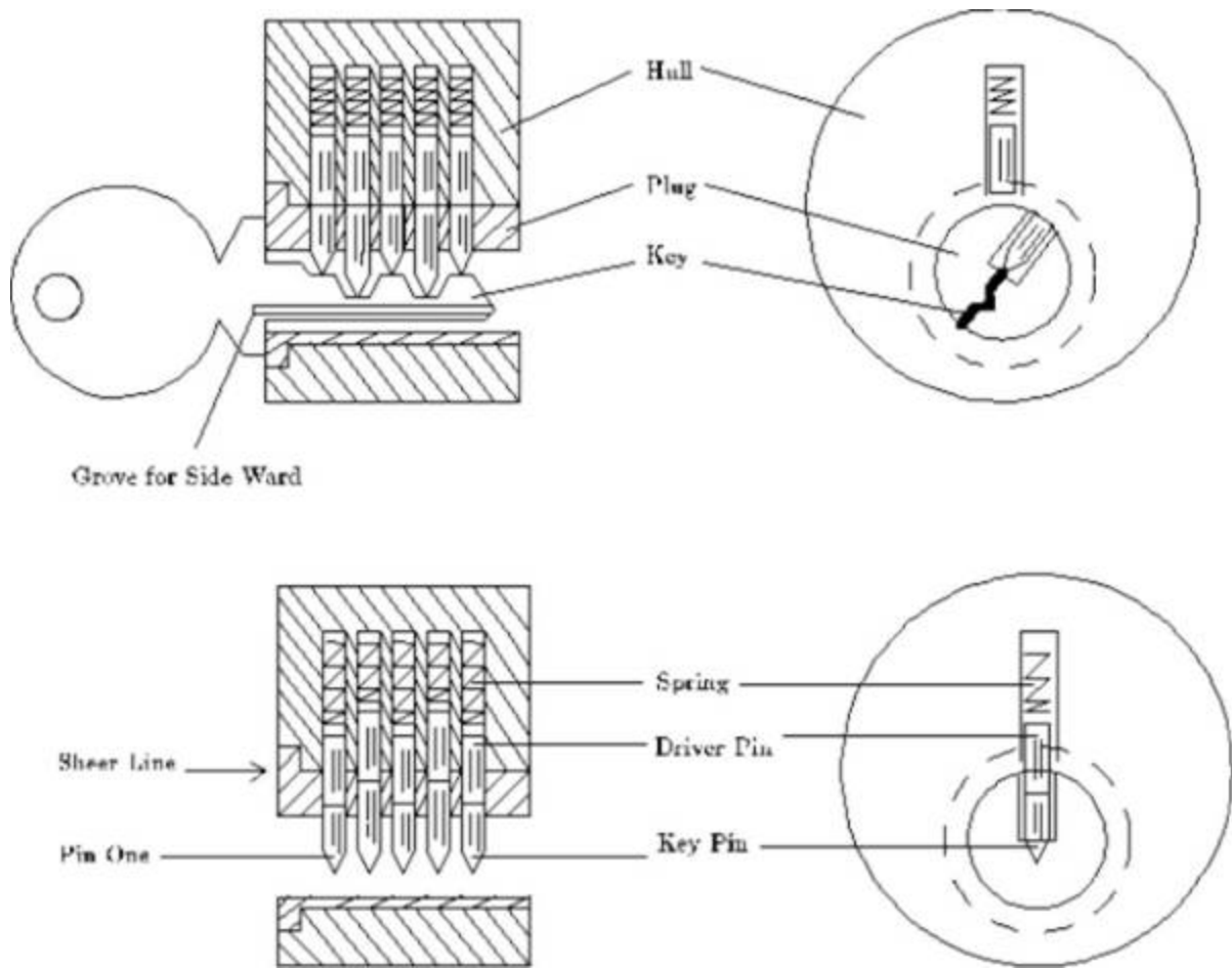
Рис. 2.1 Устройство цилиндрического замка
