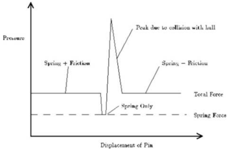
Рис. 5.5 Давление, необходимое для приведения штифтов в движение
