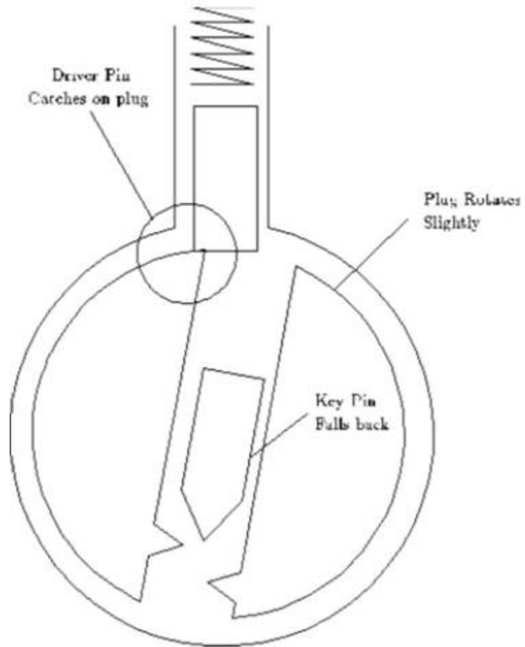
Рис. 6.1 Направляющий штифт цепляется за цилиндр
