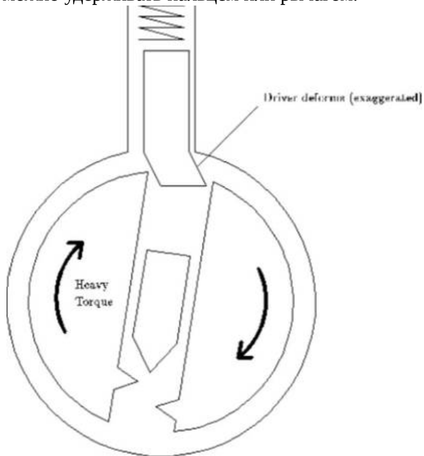
Рис. 9.2 Неправильное проталкивание направляющего штифта, вызванное эластической деформацией
