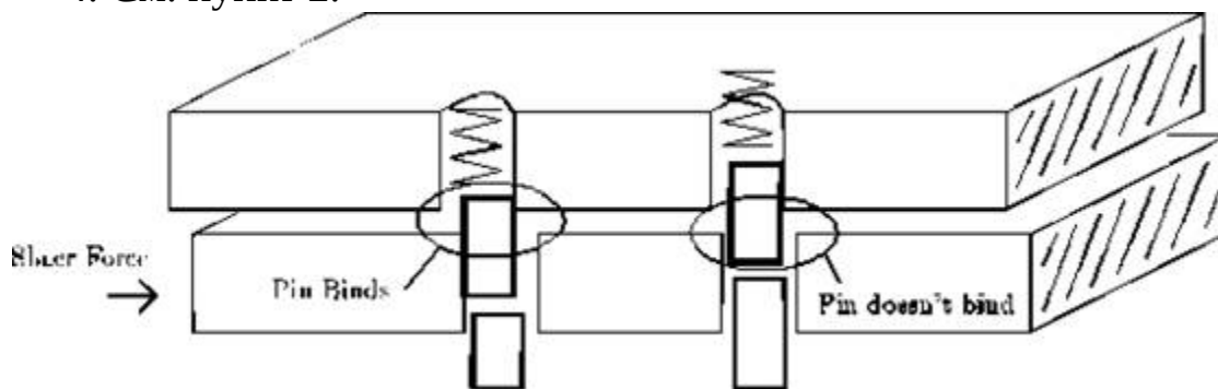
Рис. 4.1 (а) Штифт соприкасается со стенкой отверстия
