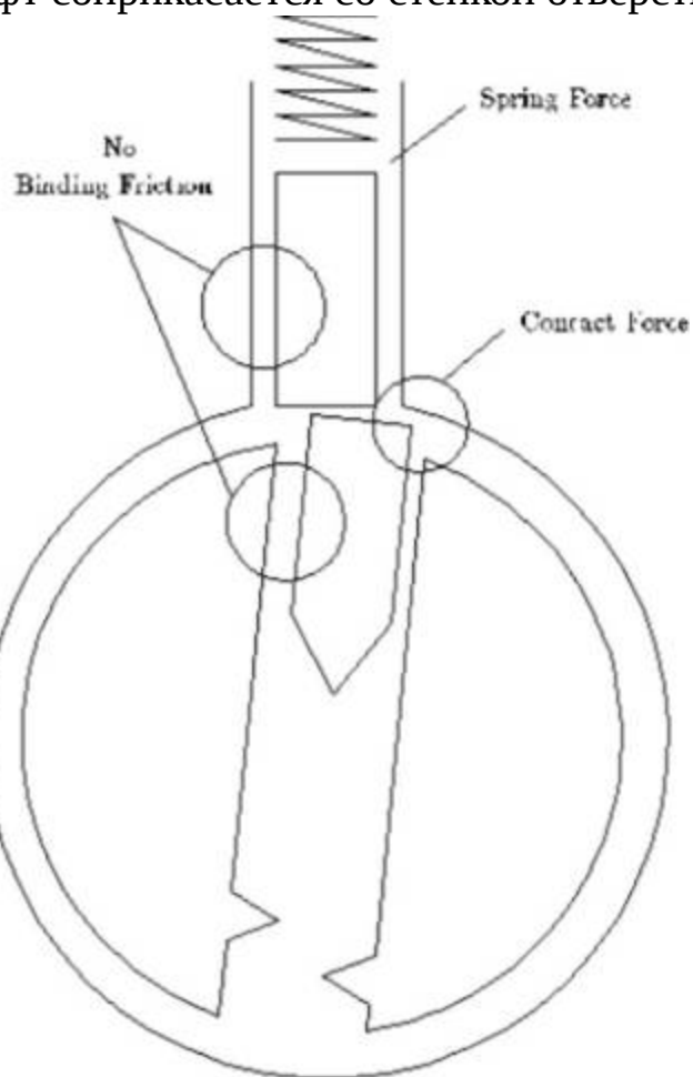
Рис. 5.3 Штифты на линии вращения
