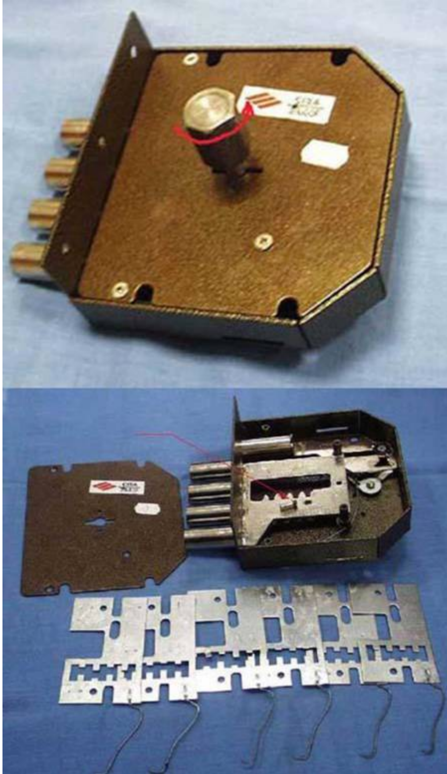
На фотографиях видна последовательность действий. Замок Cisa-Ельбор (артикул 1.06.61) подвергался воздействию свертышем на хвостовик засова. При усилнии в 10 Нм, стойка ригеля сломалась в
