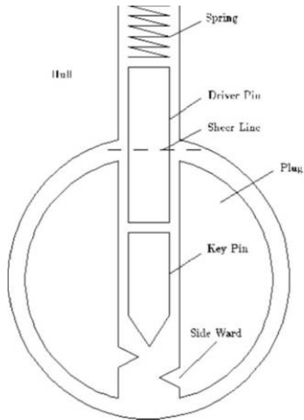
Рис. 5.1 Вертикальная модель
