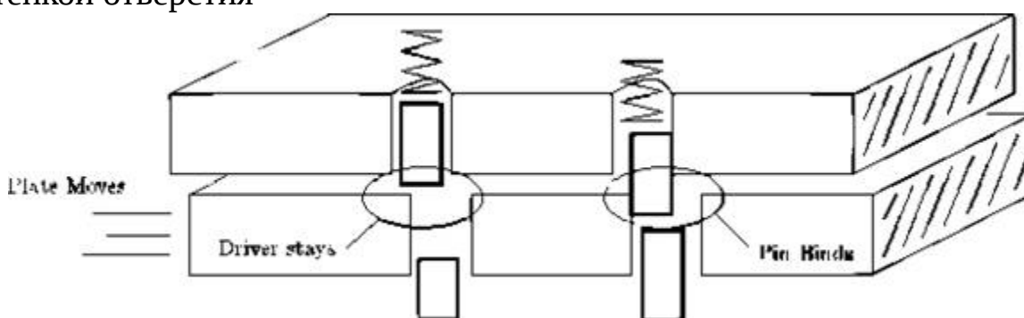
Рис. 4.3 (c) Левый направляющий протолкнут, правый соприкасается со стенкой отверстия
