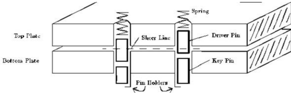
Рис. 3.1 Горизонтальная модель замка
