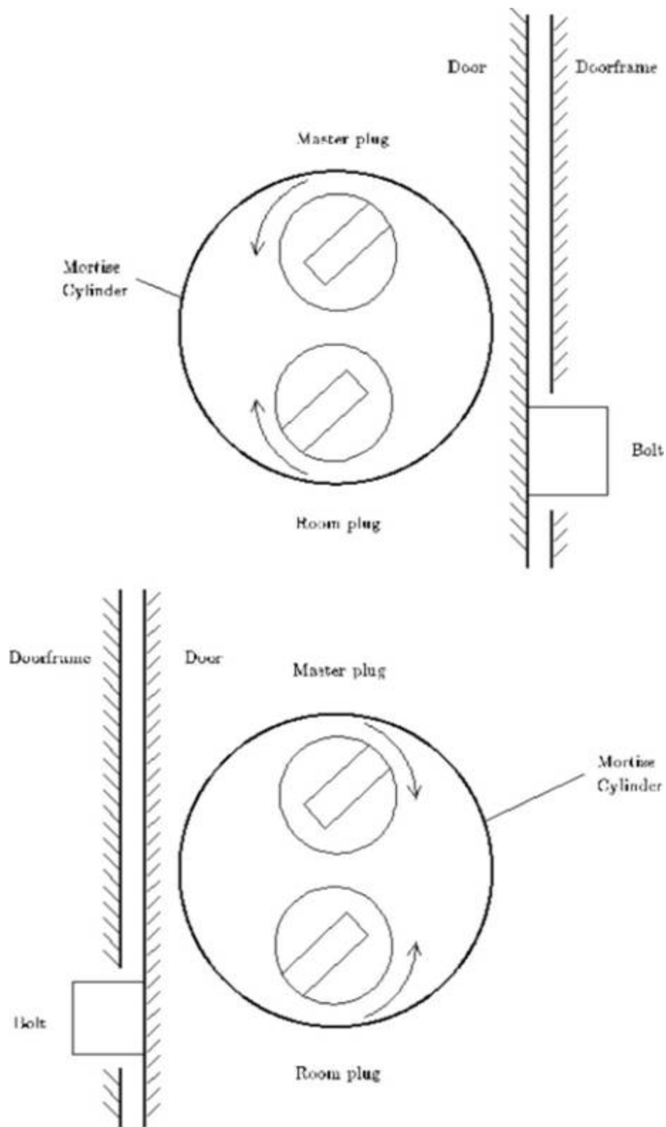
Рис. 9.1 Направление вращения цилиндра 9.2 Как далеко поворачивать
