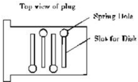
Рис. 9.10 Устройство замка с блокирующими дисками
