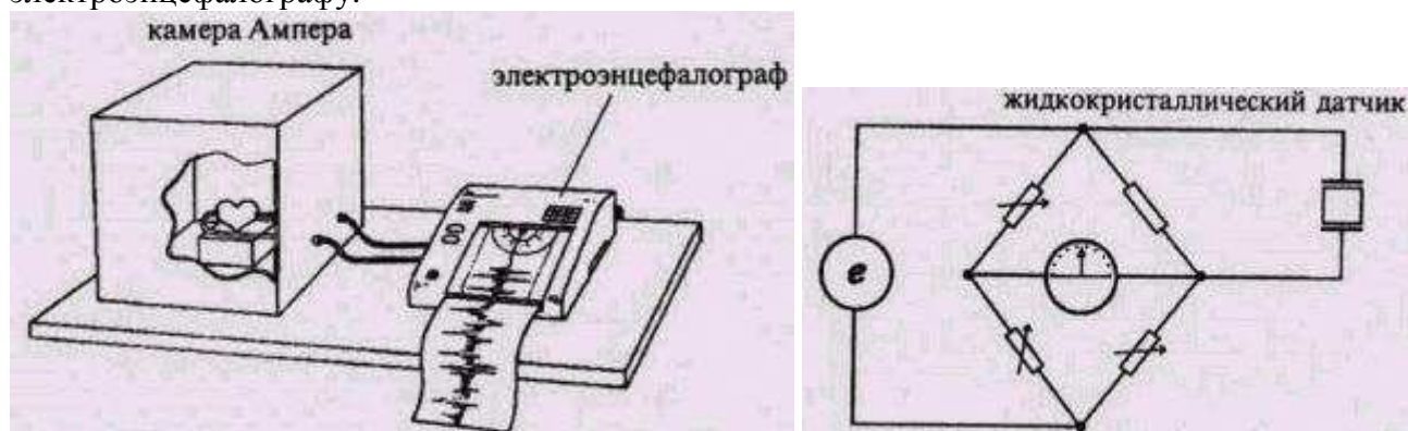
Рис. 1-8-4. Конструкция биоплазмографа.
