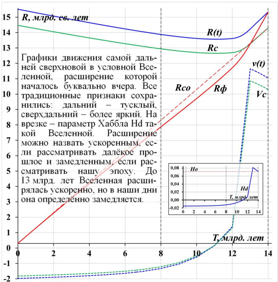
Рис.11.23. Графики движения самой дальней видимой сверхновой в замедляющейся Вселенной с параметром H_d
