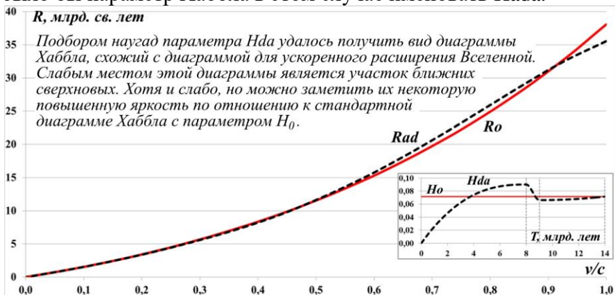
Рис.11.18. При замедленно-ускоренном расширении Вселенной с параметром H_{nd} дальние сверхновые видны более тусклыми, а сверхдальние – более яркими
