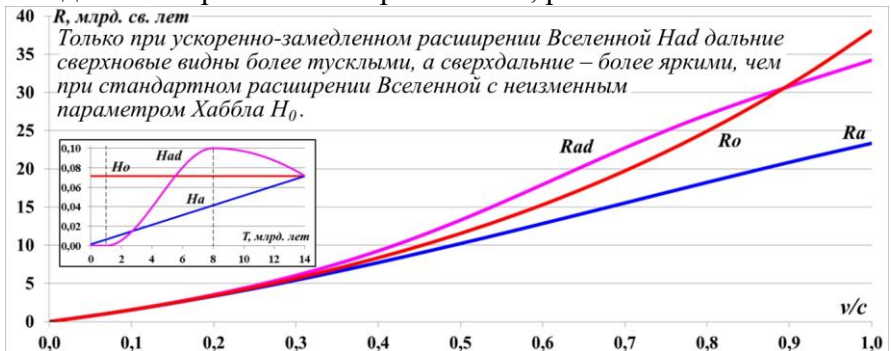
Рис.11.13. Только при ускоренно-замедленном расширении Вселенной с параметром H_{ad} дальние сверхновые видны более тусклыми, а сверхдальние – более яркими
