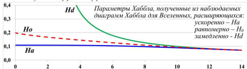
Рис.11.4. Наблюдаемые параметры Хаббла в трёх разных Вселенных.
