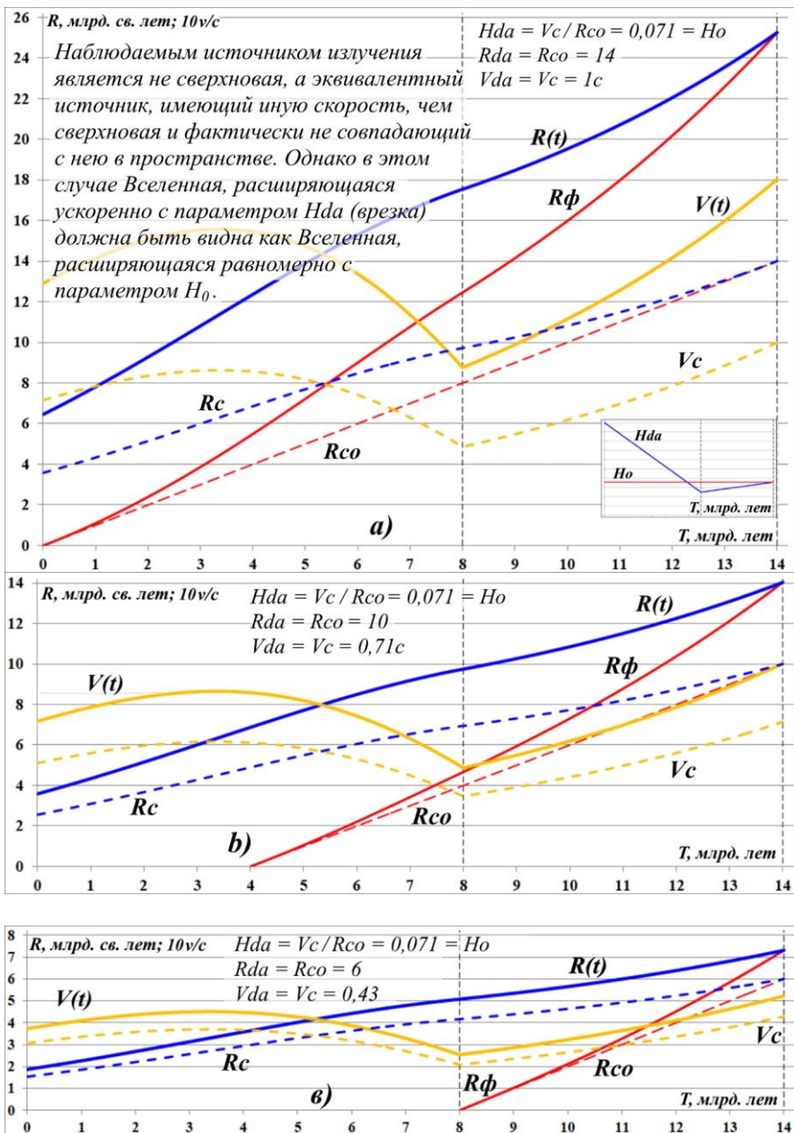
Рис.11.8. Графики движения действительного "источника" фотонов.
