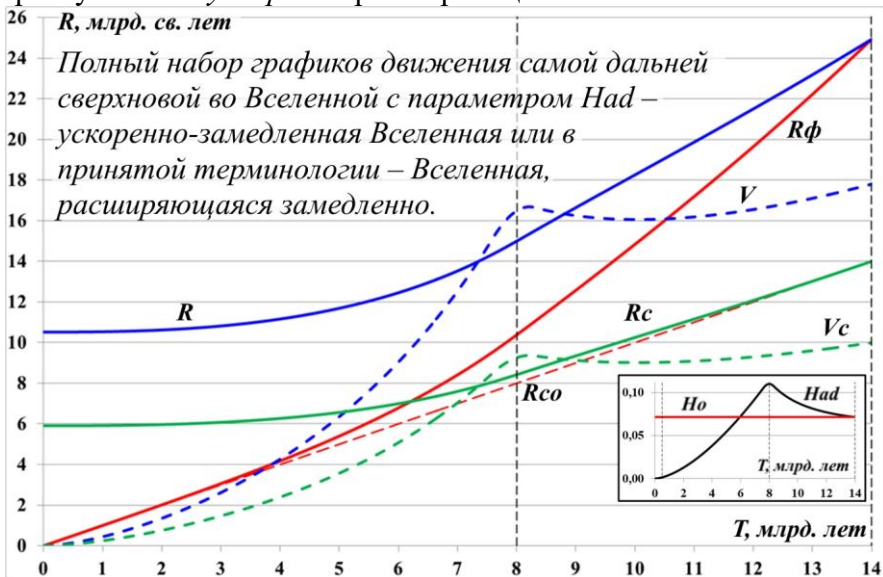
Рис.11.17. Графики движения самой дальней видимой сверхновой в замедленной Вселенной с параметром H_{ad} в виде гладкой кривой
