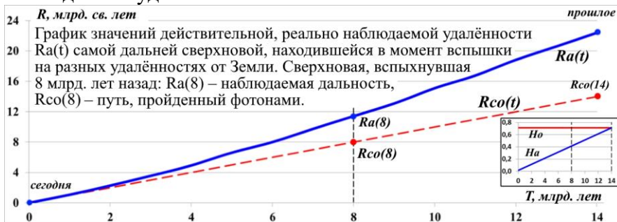
Рис.11.11. График реальной удалённости сверхновой с учётом времени в пути света от вспышки
