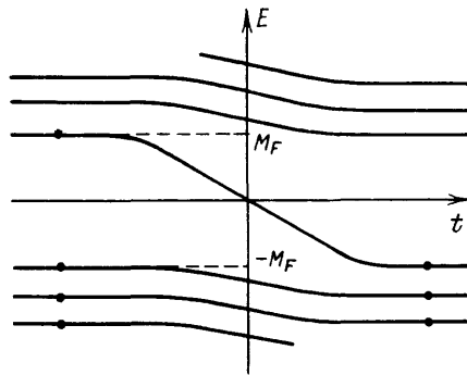
Рис. 3. Явление пересечения фермионных уровней
