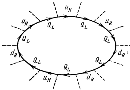
Рис. 6. Фермионная петля низшего исчезающего порядка, возникающая при описании эффектов CP-нарушения в процессах с несохранением барионного числа.
