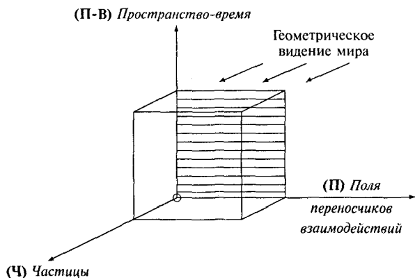
Рис. 3. Геометрическое миропонимание
