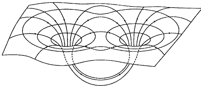
Рис. 2. Заряды в геометродинамике Уилера
