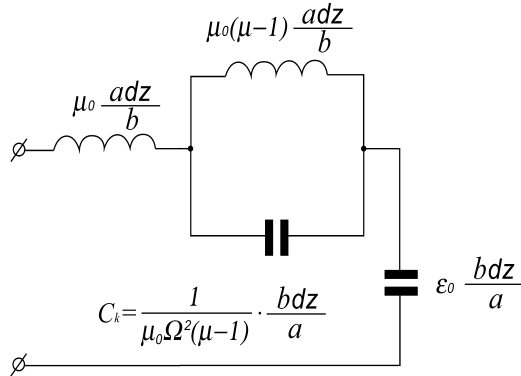
Рис. 3. Эквивалентная схема двухпроводной линии заполненной магнетиком.
