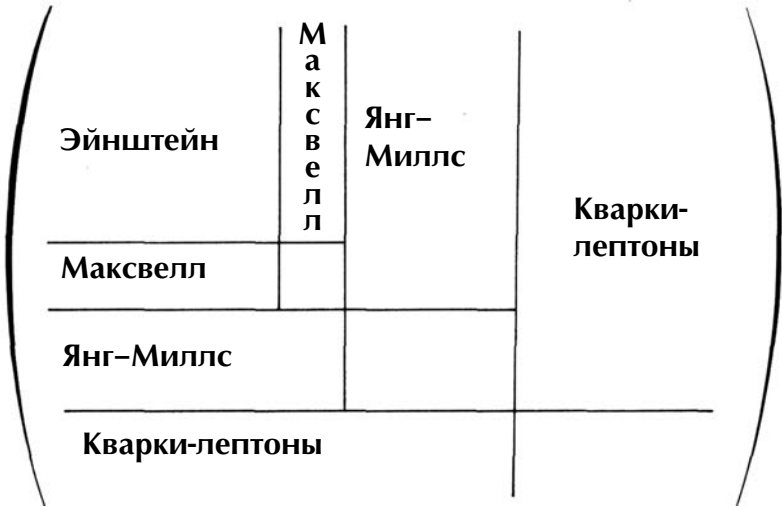
Рис. 6.3. Супергравитация — это почти воплощенная мечта Эйнштейна об исключительно геометрическом методе выведения всех взаимодействий и частиц Вселенной. Для того чтобы убедиться в этом, обратите внимание: если добавить суперсимметрию к риманову метрическому тензору, он удваивается в размерах, в итоге у нас появляется риманов метрический супертензор. Новые компоненты этого супертензора соответствуют кваркам и лептонам. Разделяя риманов супертензор на компоненты, мы обнаружим, что он содержит почти все элементарные частицы и взаимодействия, какие есть в природе: теорию гравитации Эйнштейна, поля Янга-Миллса и Максвелла, кварки и лептоны. Но, поскольку в этой картине отсутствуют конкретные частицы, мы вынуждены обратиться к более эффективному набору формул — к теории суперструн
