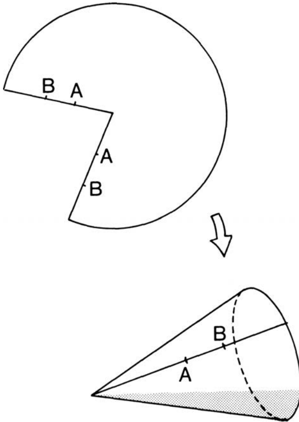
Рис. 9.3. Если мы соединим точки A и B , то получим конус — простейший пример орбиобразия. В теории струн наша четырехмерная Вселенная может иметь шестимерную пару с топологией орбиобразия. Однако шестимерная Вселенная так мала, что не поддается непосредственному наблюдению
