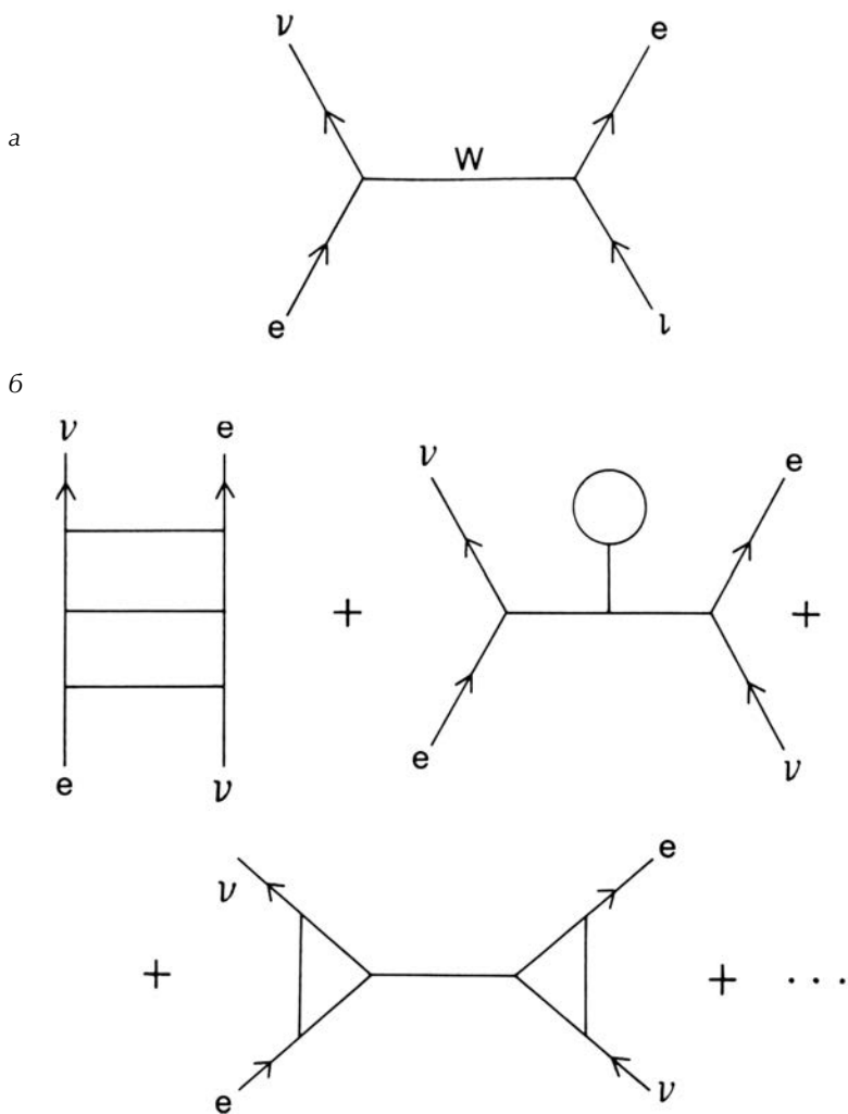
Рис. 5.2. а — по квантовой теории при столкновении субатомные частицы обмениваются порциями энергии, или квантами; электроны и нейтрино обмениваются квантом слабого взаимодействия, называемым W -частицей; б — для вычисления полного взаимодействия электронов и нейтрино необходимо добавить бесконечный ряд линий — диаграмм Фейнмана, на которых обмен квантами представлен в виде постепенно усложняющихся геометрических рисунков. Этот процесс добавления бесконечного ряда линий к диаграммам Фейнмана называется теорией возмущений
