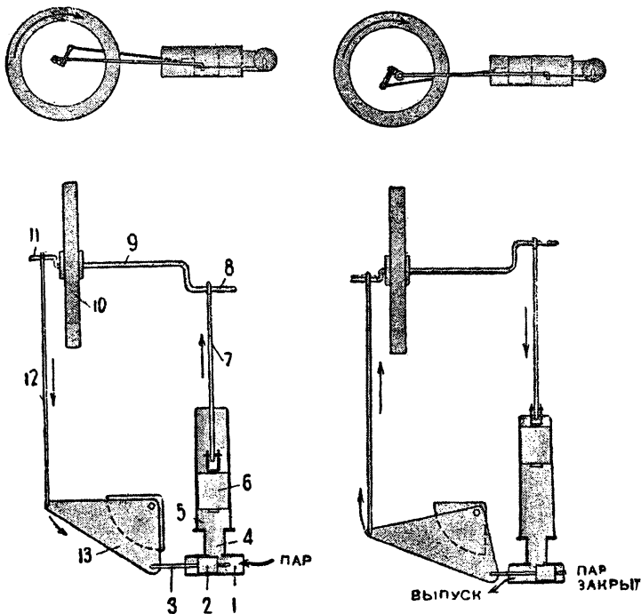
Рис. 84. Наверху — схема работы одноцилиндровой машины (вид сбоку), внизу — вид машины сверху: 1 — трубка золотника, 2 — поршень, 3 — шток золотника, 4 — соединительная трубочка, 5 — цилиндр машины, 6 — поршень, 7 — шатун поршня, 8 — кривошип вала, 9 — вал, 10 — маховое колесо, 11 — второй кривошип, 12 — тяга треугольника, 13 — треугольник.
