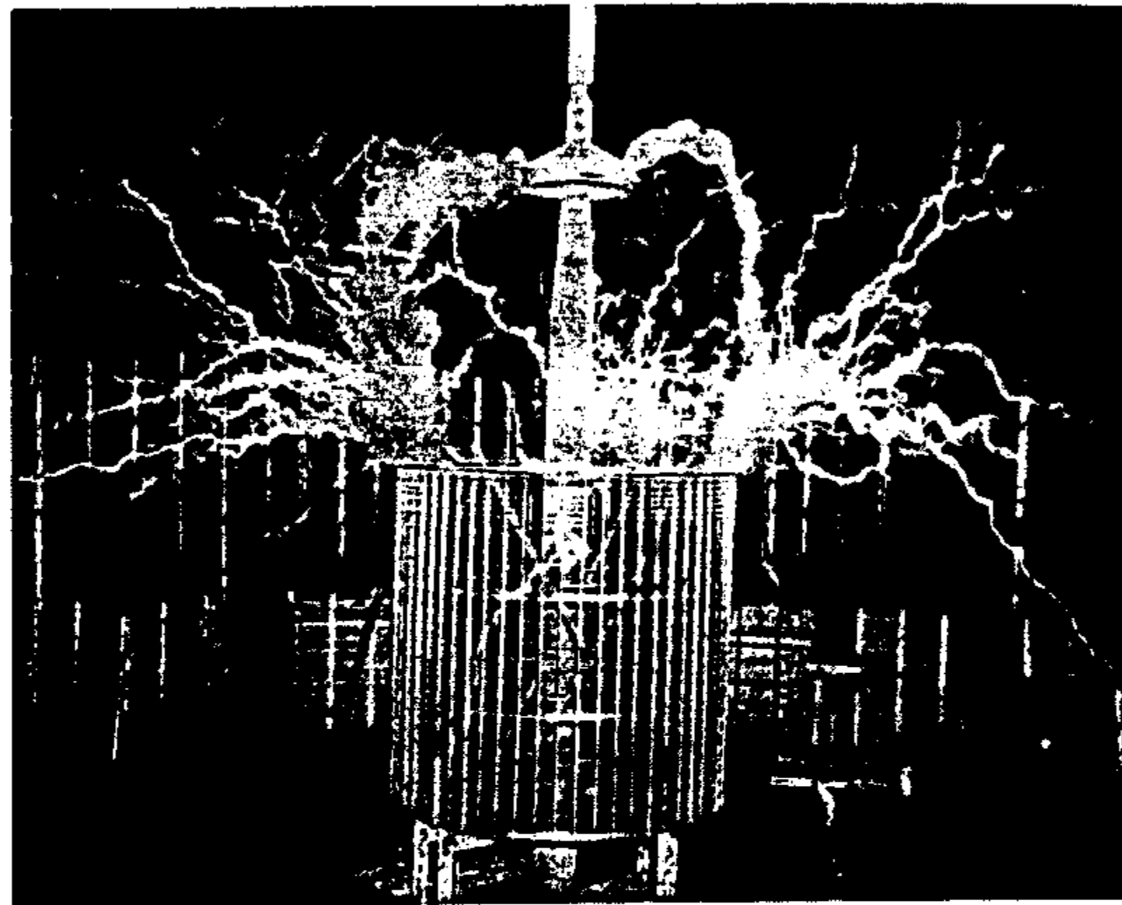
Фото LIII. Условия выброса разряда подобны тем, что на фото LII, при однократном замыкании цепи, но на более длительный промежуток времени
