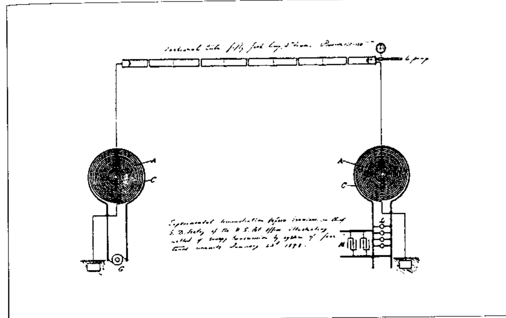
Ил. 1. Схема устройства, осуществляющего передачу электрической энергии через разреженный газ (подлинный диапозитив Теслы из Музея Николая Теслы в Белграде). Демонстрация опыта в присутствии главного эксперта (фамилия – неразборчиво) из Патентного ведомства США с целью иллюстрации метода передачи энергии с помощью системы четырех резонансных контуров. 23 января 1898 года
