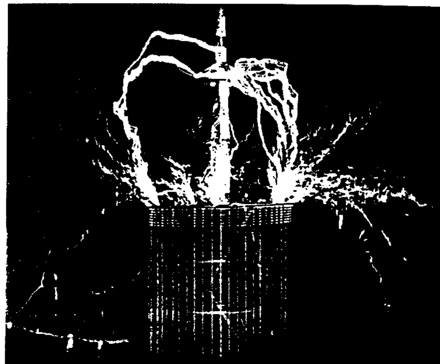
Фото VI. Нормально возбужденная экстра-катушка
