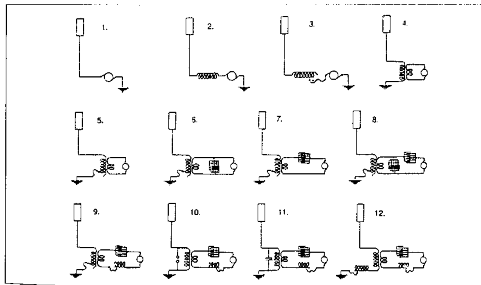
Ил. 3. Способы подключения генератора переменного тока к системе «Антенна – земля» (подлинный диапозитив Теслы)
