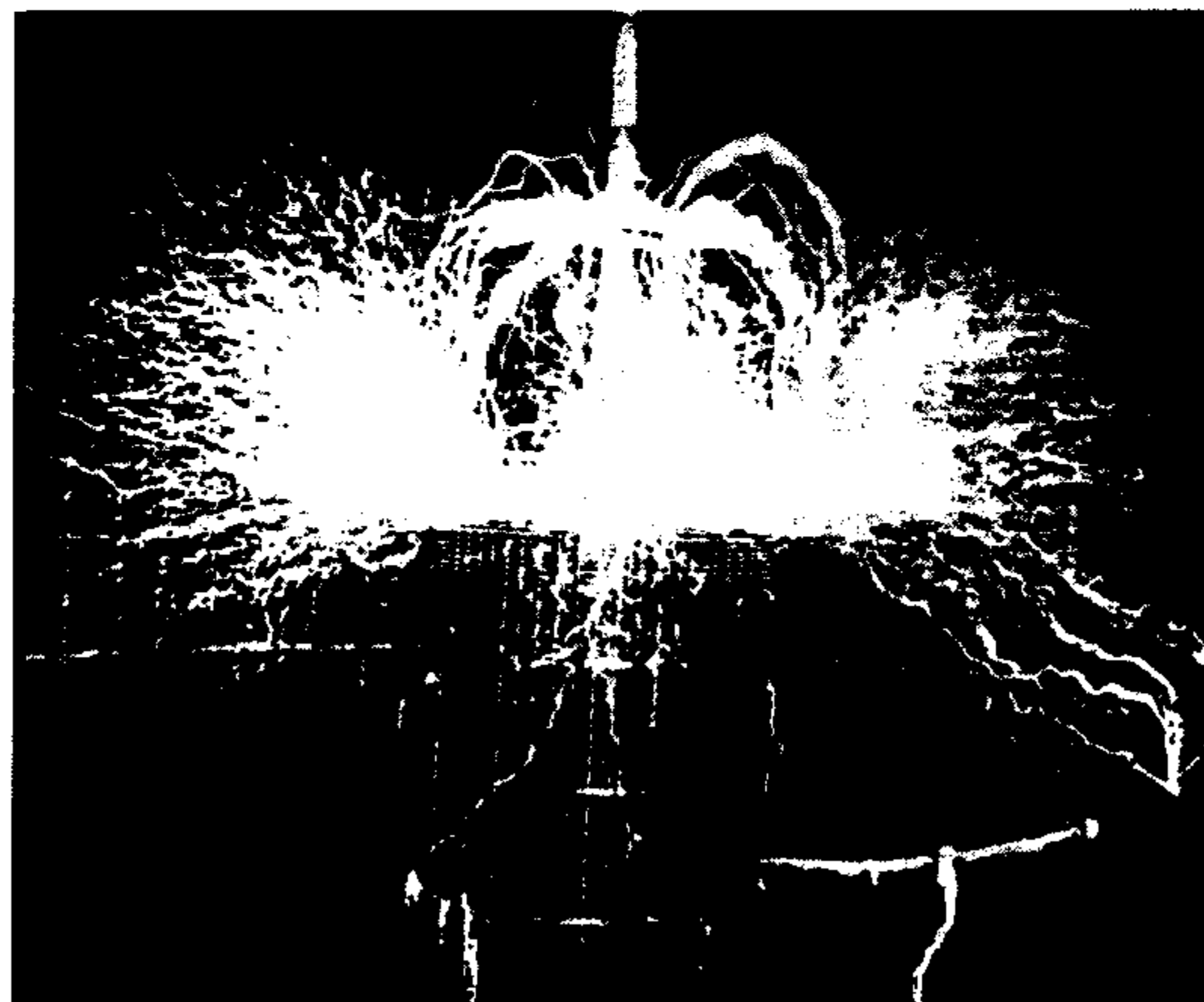
Фото X. Разряд, исходящий от латунного кольца на вершине экстра катушки
