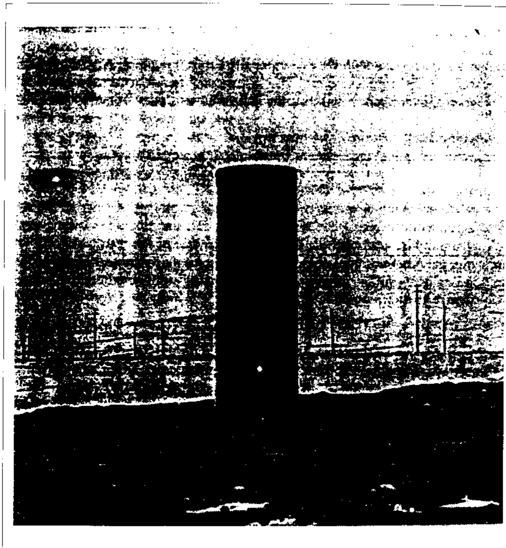
Фото XXV. Катушка за пределами лаборатории, ее нижний конец соединен с заземлением и со свободным верхним концом. Свечение лампы вызвано током, индуцированным в трех витках провода, намотанного вокруг нижнего конца катушки
