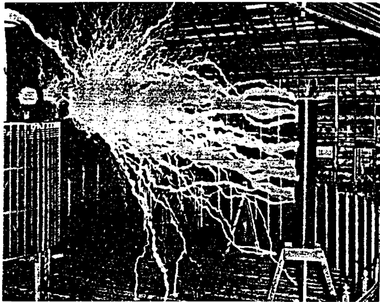
Фото XI. Разряд, идущий буквально на фотокамеру, от центральной катушки к другой, расположенной на штативе. М-р Алли сидит на стуле
