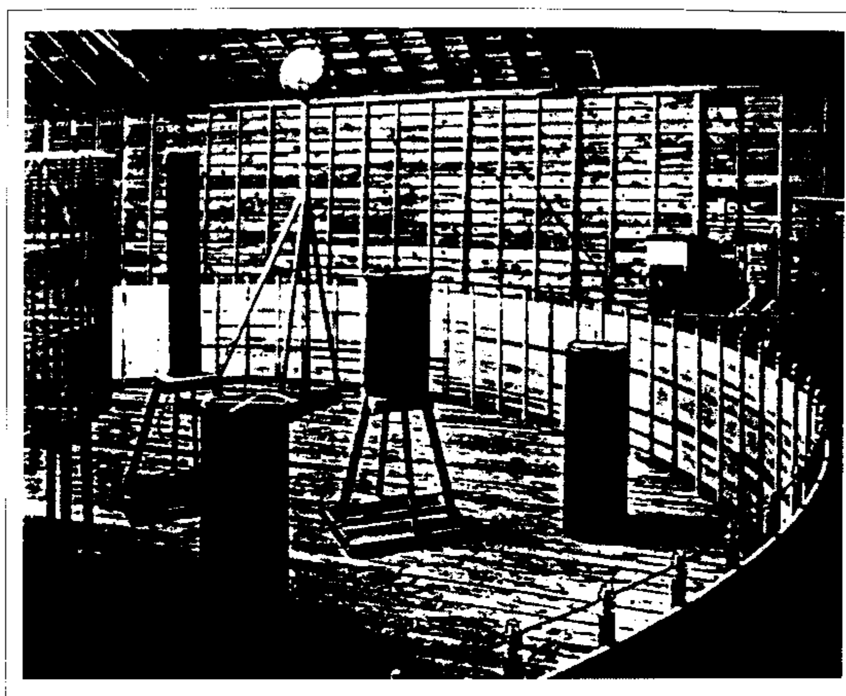
Фото II. Внутренний вид помещения. Половина круглого каркаса генератора колебаний и несколько катушек внутри него
