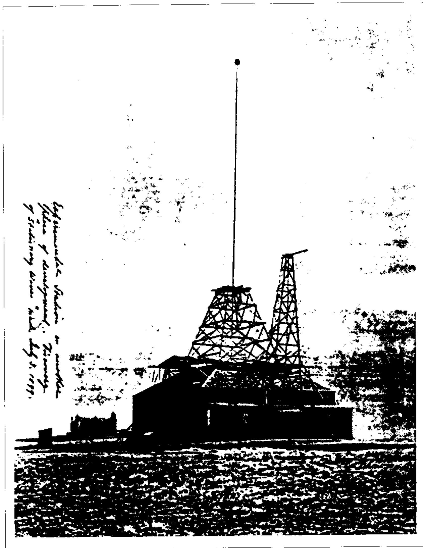
Фото I. Лаборатория. Вид спереди со склона Пайкс-Пик Текст на фото: Экспериментальная станция в фазе становления. Открытие стоячих волн, состоявшееся 9 июля 1899 г.
