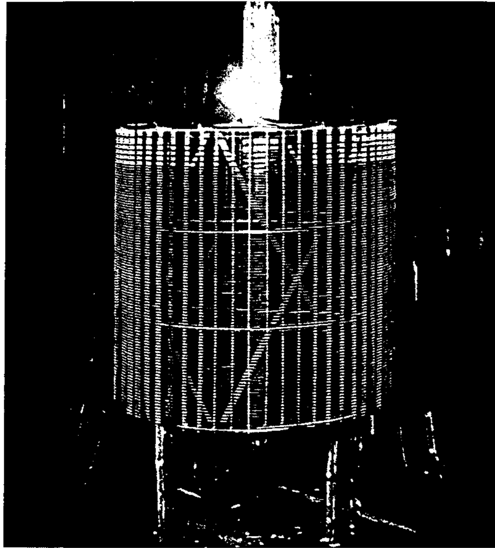
Фото XXVIII. Лампа накаливания в состоянии свечения под воздействием тока, идущего от экстра-катушки к конструкции из стальных труб.
