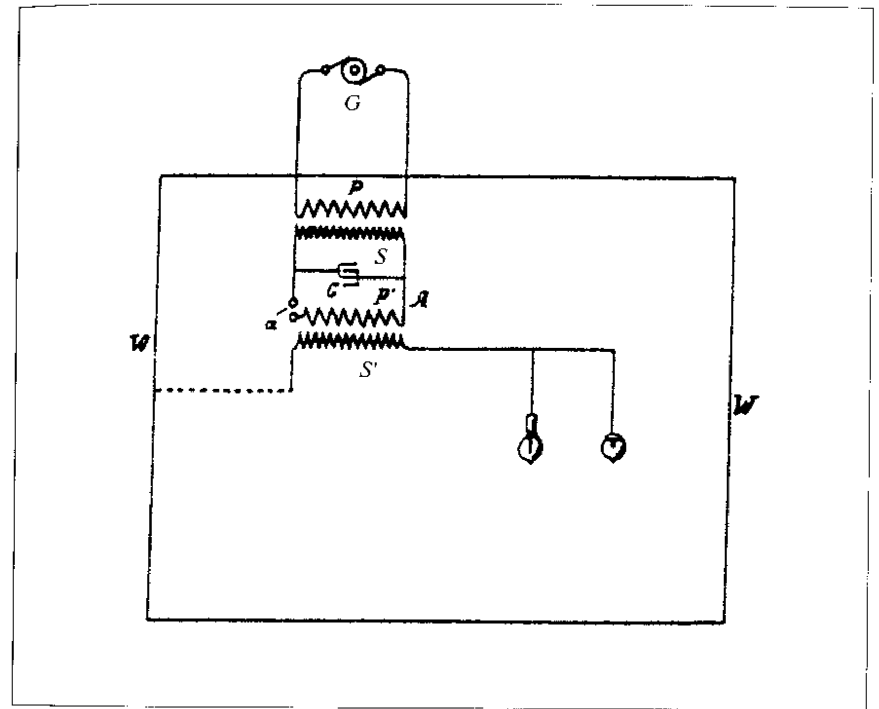
Ил. 2. Установка для электрического освещения
