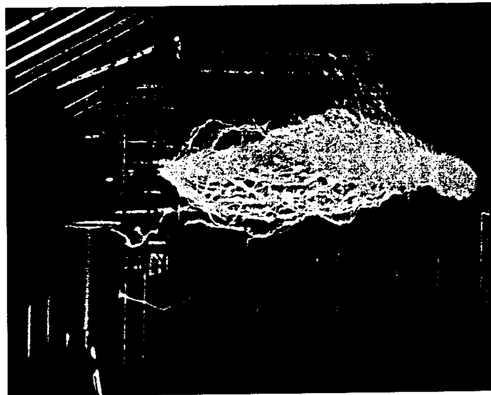
Фото LVI. Разряд экстра-катушки, который исходит от шара диаметром 30", являющегося свободным выводом, к катушке на подставке
