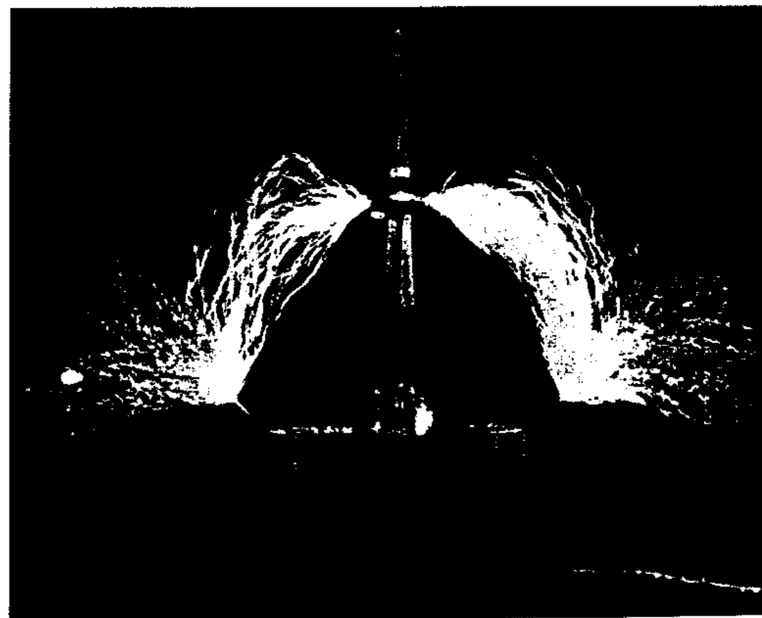
Фото LVIII. Разряд от экстра-катушки, исходящий от двух диаметрально расположенных проводов, направленных вверх и закрепленных на латинном кольце на верхи катушки
