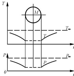
Рис. 4.17. Распределение температуры и давления вокруг совокупности торональных вихрей в свободном пространстве
