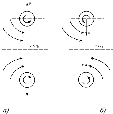
Рис. 1.3. Взаимодействие двух цилиндрических газовых вихрей:
