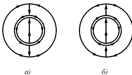
Рис. 2.2. Образование присоединенного вихря: a – при увлечении прилегающих к основному вихрю слоев газа; б – при делении основного вихря
