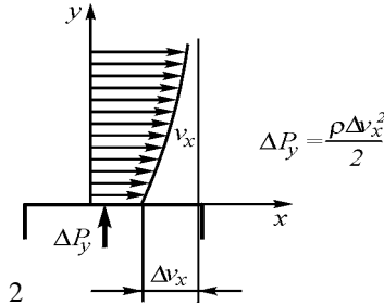
Рис. 4.22. Происхождение поперечной силы, действующей на поверхность тела со стороны омывающего потока
