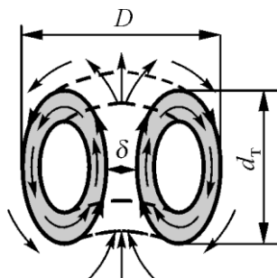
Рис. 4.13. Торoidalный газовый вихрь в разрезе
