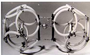
7.2.2. Модель 2\text{H}_2\text{O}
