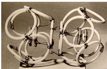
6.2.4. Модель молекулы F 2
