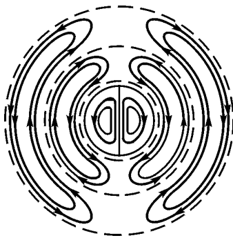
Рис. 2.3. Вихрь Тэйлора
