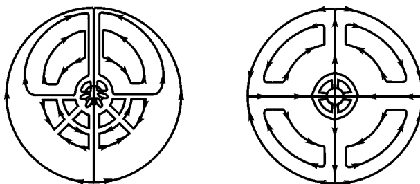
Рис. 2.7. Структура атома бериллия
