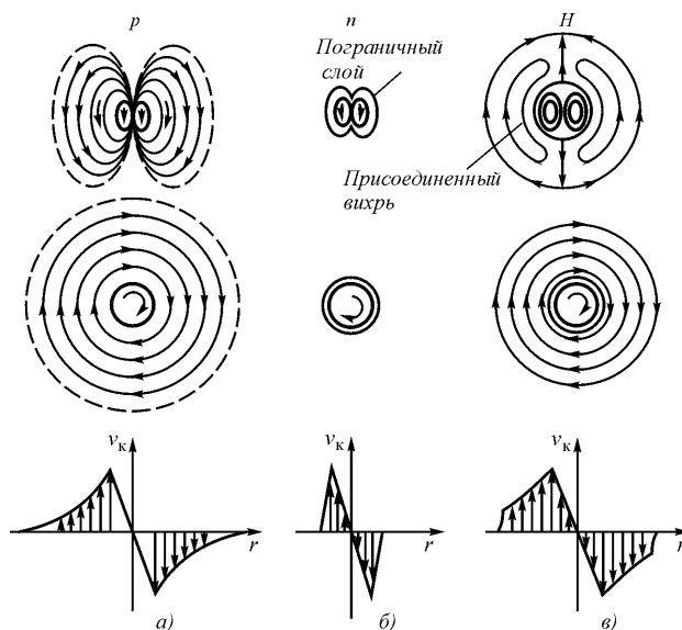
Рис. 2.1. Три устойчивых состояния протона: а – собственно протон; б – нейтрон; в – атом водорода
