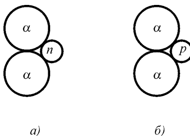
Рис. 1.12. Обеспечение стабильности изотопа атома бериллия {}_4\text{Be}^9 и {}_5\text{B}^9 .
