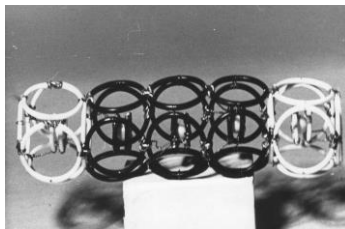
7.2.16. Модель молекулы C_3O_2
