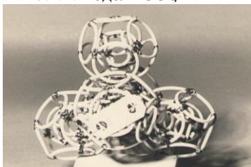
7.4.3. Модель молекулы PCl_5
