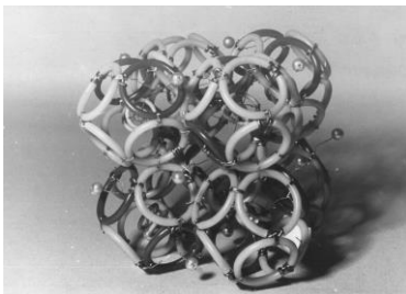
7.2.4. Модель 8\text{H}_2\text{O}
