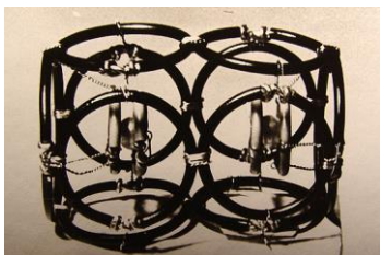
6.2.3. Модель молекулы N 2
