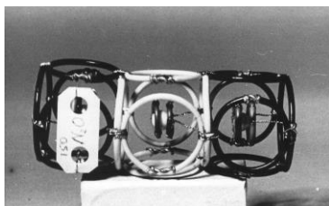
7.2.15. Модель молекулы N_2O
