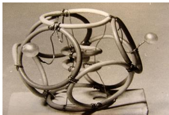
7.3.2. Модель молекулы NH_3
