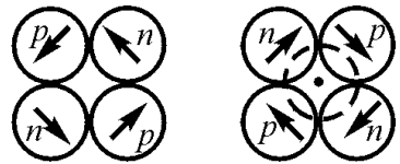
Рис. 1.17. Структура ядра ^4\text{Be}^9
