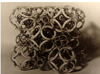
6.5.4. Модель NaCl
