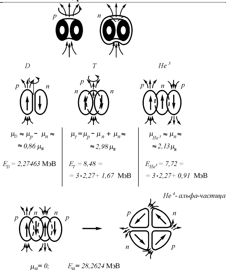
Рис. 1.11. Структура протона (а), нейтрона(б), дейтрона (в), тритона (з), ядра гелия-3 (д) и ядра гелия-4 – альфа частица (е)
