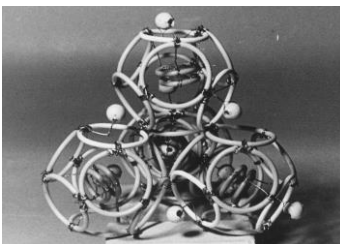
7.1.5. Модель молекулы \text{BH}_4^- 7.1.6. Модель молекулы \text{Be}(\text{H}_2\text{O})_4^{2+} Модели соединений кислорода
