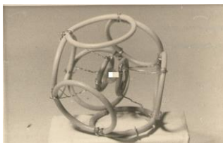
5.2.5. Модель атома углерода
