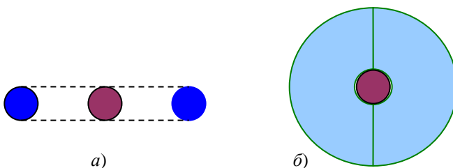
Распределение материи в атоме водорода: a) по Огжевальскому; б) по эфиродинамике.
