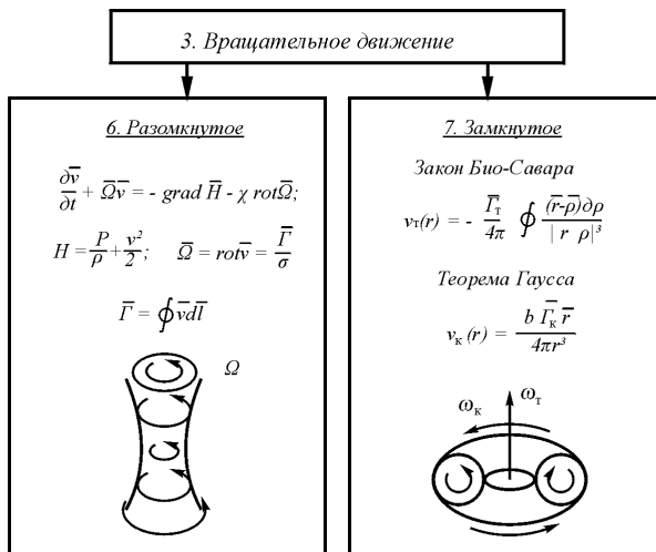
Рис. 3.4. Вращательная форма движения эфира
