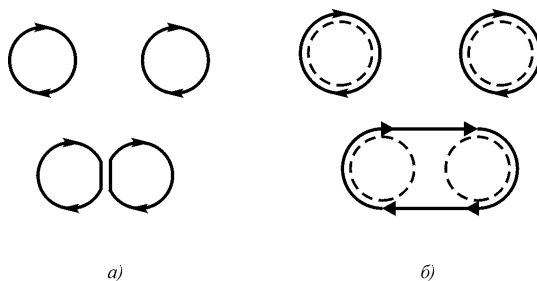
Рис. 3.1. Соединение вихрей: a – путем прилипания друг к другу (соответствует ионной связи); б – путем образования общих потоков (соответствует ковалентной связи)
