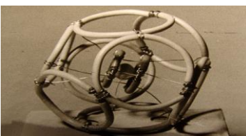
5.2.6. Модель атома хлора
