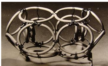
6.2.2. Модель молекулы O 2
