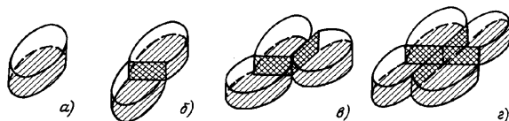
Рис. 1.13. К объяснению периодичности приращения энергии связей нуклонов при наращивании числа нуклонов в ядре: установка на поверхности ядра одного (а), двух (б), трех (в) и четырех (г) нуклонов.
