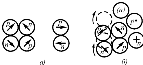
Рис. 6.15. Структура ядра {}^7_3\text{Li}
