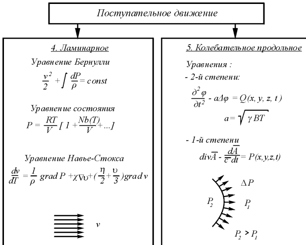
Рис. 3.3. Поступательная форма движения эфира
