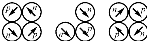
Рис. 1.21. Структура ядра {}_5\text{B}^{11}
