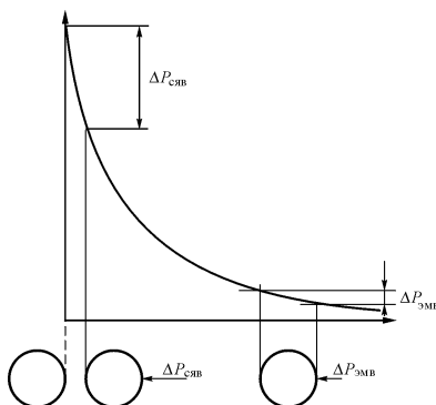
Рис. 1.5. Взаимодействие частиц вещества через градиенты давлений
