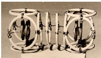
6.2.5. Модель молекулы O 2
