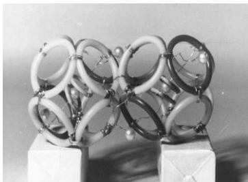
7.2.3. Модель 4\text{H}_2\text{O}
