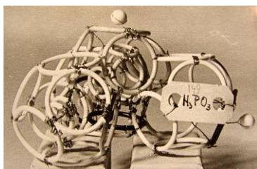
7.2.19. Модель молекулы H_3PO_3
