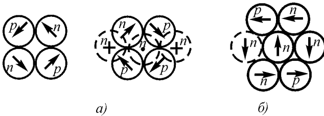
Рис. 1.18. Структура ядер ^4\text{Be}^{10} (а) и ^4\text{Be}^{11} (б)
