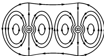
Рис. 3.2. Образование молекулы H_2
