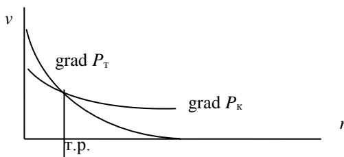
Рис. 1.9. Распределение градиентов давлений эфира вблизи поверхности нуклона; т.р. — точка равновесия давлений
