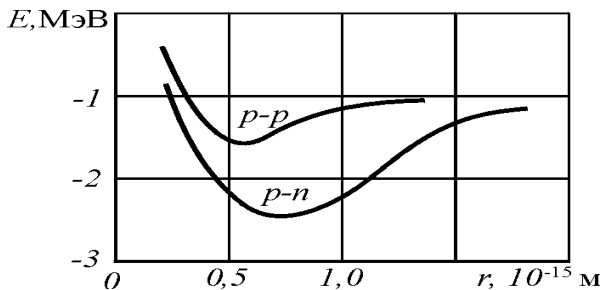
Рис. 1.6. Зависимость энергии взаимодействия между нуклонами (протон-протонное и протон-нейтронное взаимодействия) от расстояния между ними при антипараллельных спинах
