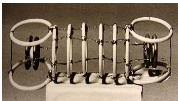
6.2.6. Модель молекулы N 2 модификация пар
