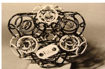
7.2.18. Модель молекулы P_4O_6
