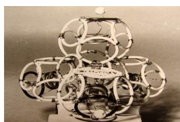
7.2.20. Модель молекулы H_3PO_4
