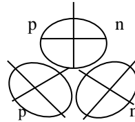
Рис. 1.23. Структура ядра 6C^{12}
