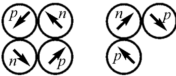
Рис. 1.16. Структура ядра ^4\text{Be}^7
