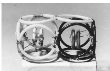
7.2.13. Модель молекулы \text{C-O}^+
