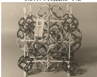
6.5.3. Модель CaTiO 3
