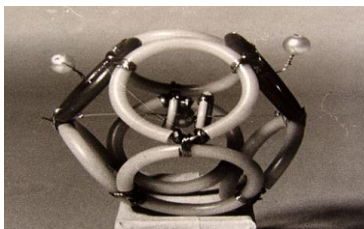
7.2.1. Модель молекулы \text{H}_2\text{O}
