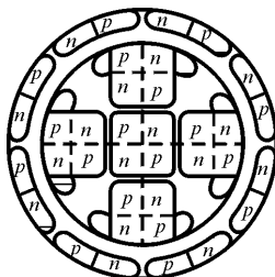
Рис. 1.27. Структура ядра {}_{64}\text{Gd}^{146} .
