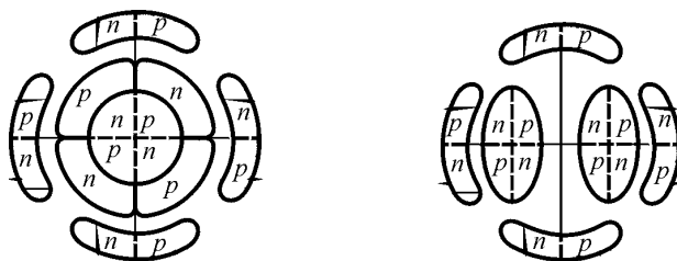
Рис. 1.25. Структура ядра {}^{20}\text{Ca}^{40}
