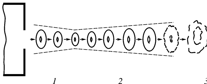
Рис. 4.18. Движение и преобразование газового тороида: 1 – стадия сжатия тороида; 2 – стадия расширения тороида (диффузия); 3 – стадия развала тороида.
