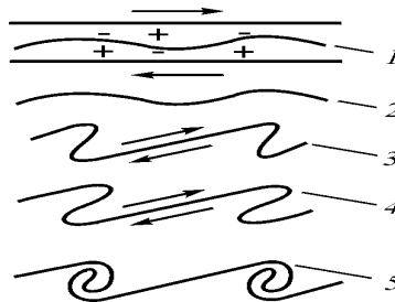
Рис. 4.10. Неустойчивость пограничного слоя между потоками газа: стрелками указаны направления течений; области повышенного давления обозначены знаками +, цифры соответствуют стадиям развития процесса
