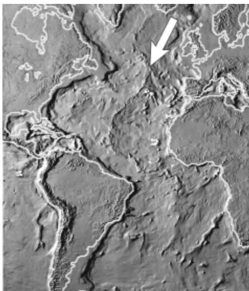
Срединно-Атлантический хребет (стрелка) ясно виден на фотографии, сделанной со спутника
