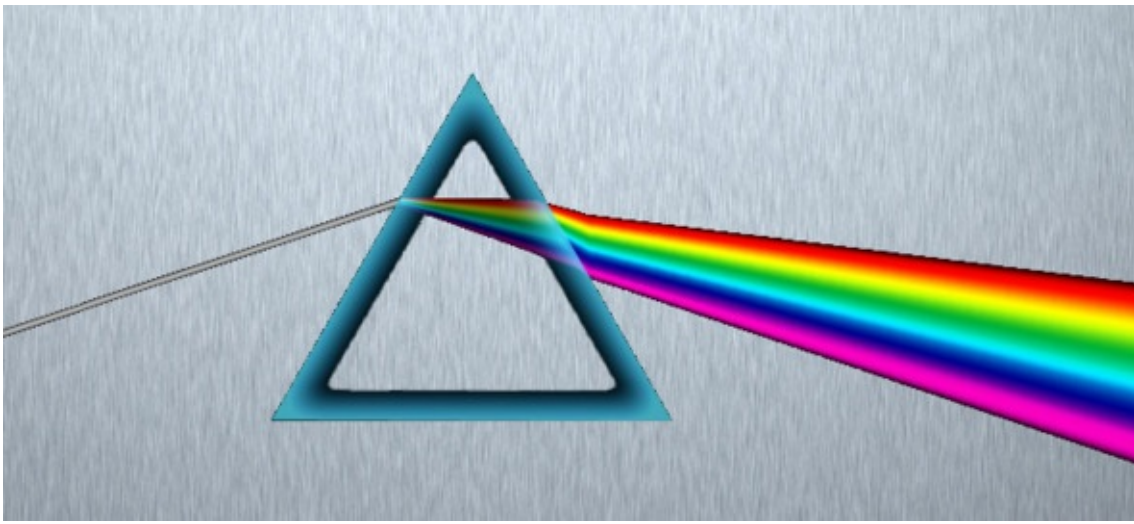
Дисперсия информации.
