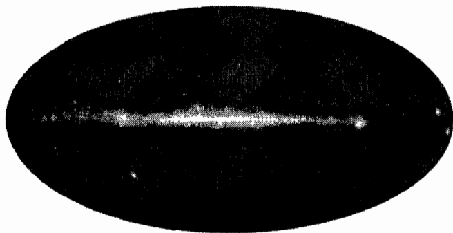
Рис. 70. Микроволновое излучение
