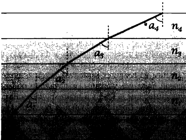
Рис. 17. Оптико-механическая аналогия
