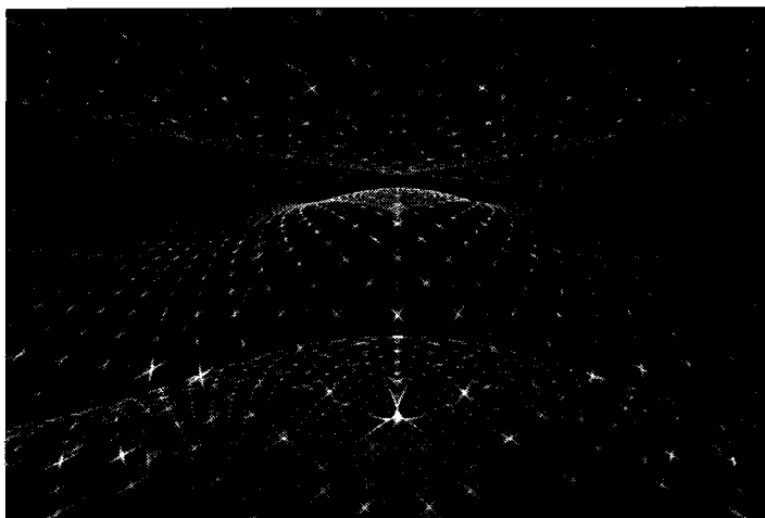
Рис. 63. Квантовая флуктуация
