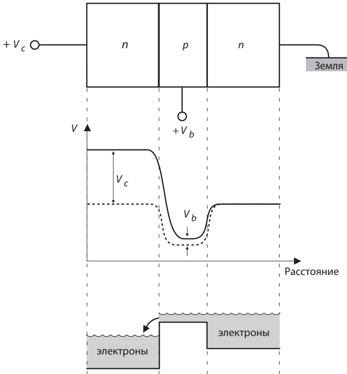
Рис. 9.4. Транзистор
