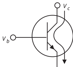
Рис. 9.5. Аналогия транзистора с водяными трубками
