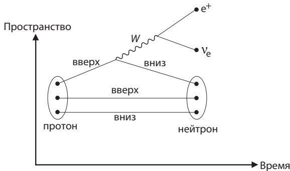
Рис. 11.3. Превращение протона в нейтрон в рамках слабого взаимодействия с испусканием позитрона и нейтрино.
