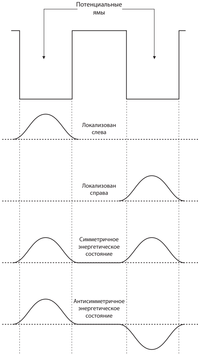
Рис. 8.1. Сверху изображен двухямный потенциал, а снизу — четыре интересные волновые функции, описывающие электрон в этом потенциале. Только две нижние функции соответствуют электрону с определенной энергией
