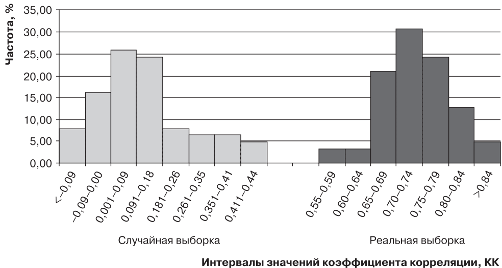
Рис. 5.4. Гистограммы распределения КК между половинами теста MADRS в реальной и случайной выборках
