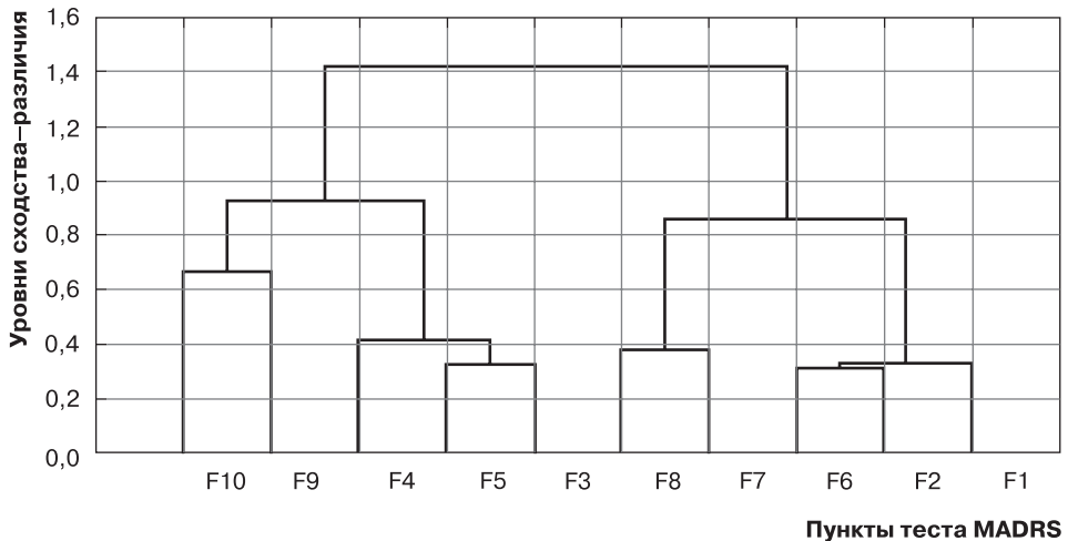
Рис. 5.5. Иерархическая дендрограмма сходства – различия между пунктами теста MADRS
