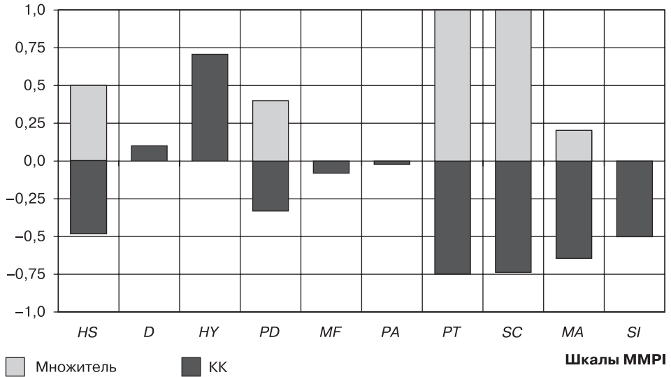
Рис. 5.3. Сопоставление значений поправочных множителей и коэффициентов корреляции (КК)
