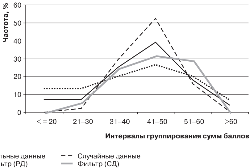
Рис. 5.2. Распределение сумм баллов по тесту MADRS
