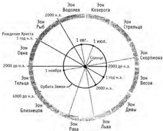
Рисунок 1. Прецессия равноденствий.
