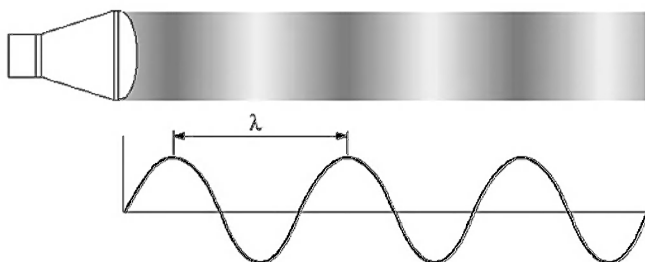
Рис. 1. Плотности в ультразвуковой волне (Митьков В.В., 2005)
