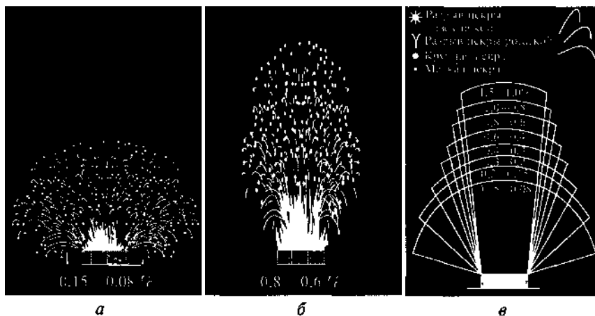
Рис. 8. Образцы «горячей пробы», в которой по характеру столба искр при пробном разливе сплава сталевар определял процентное содержание углерода 1
