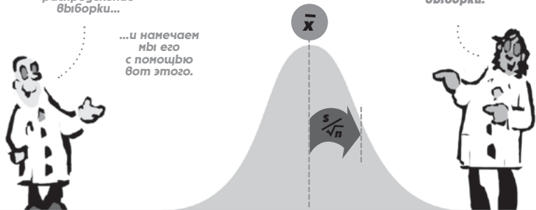
Предполагаемое распределение всех возможных значений \bar{x}
