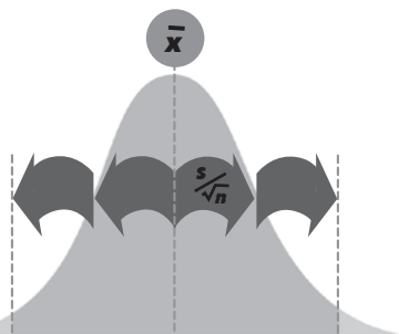
Предполагаемое распределение выборки для \bar{x}
