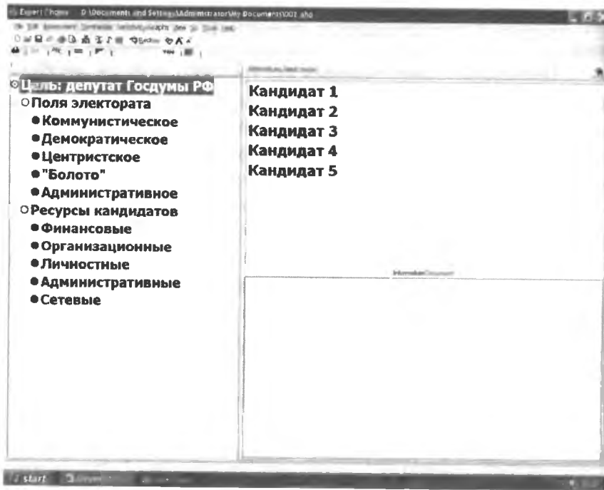
Рис. 3.1. Модель избирательного процесса
