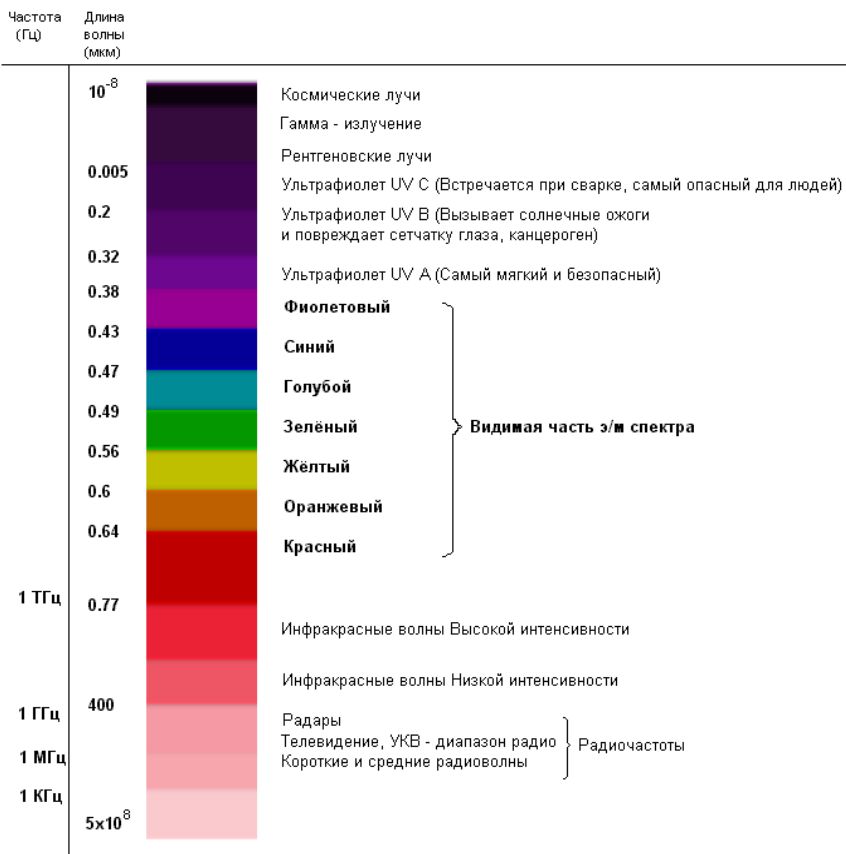
Рис. 3. Шкала элеткромагнитного излучения
