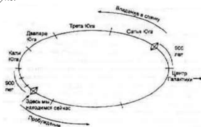
Рис Сверхбольшие циклы в индийских учениях.
