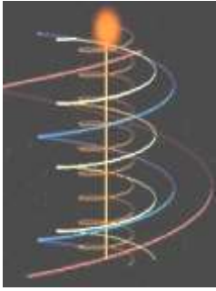
Движение планет Солнечной системы
