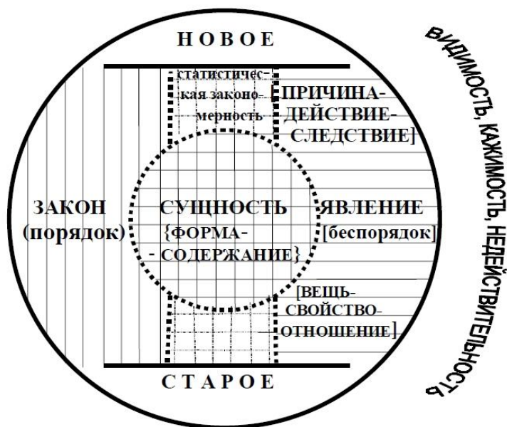
Рис. 18. Диаграмма (структурная схема) категории “действительность”
