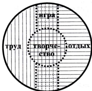
Рис. 28. Диаграмма «Формы человеческой деятельности»
