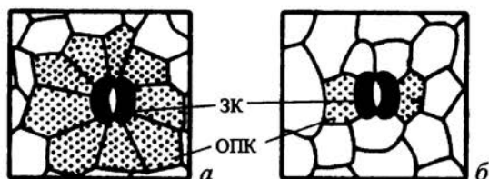
Рис. 76. Отдел Cycadophyta (C 2 —Q).
