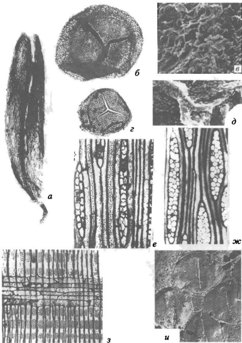
Рис. 53. Отдел Archaeopteridophyta ( D_3-C_1 ); роды Archaeopteris (a—д) и Callixylon (e—и):
