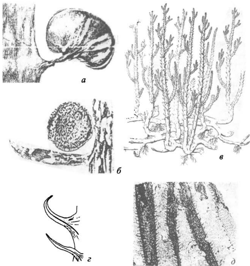
Рис. 14. Класс Lycopodiopsida (D—Q).
