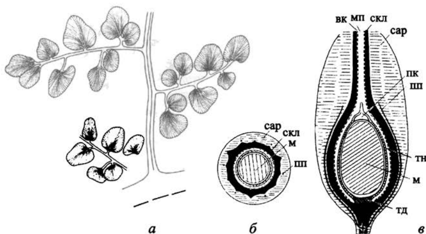
Рис. 65. Отдел Lyginopteridophyta ( D_3-K_1 )
