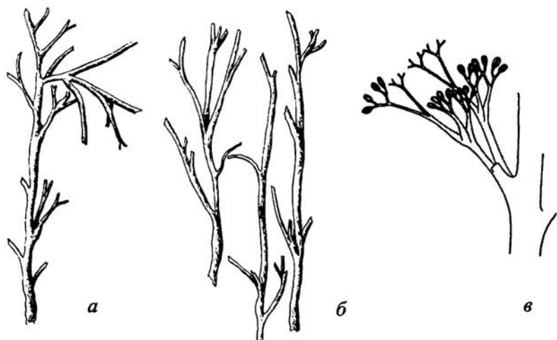
Рис. 7. Класс Rhyniopsida ( S_1-D_2 ).
