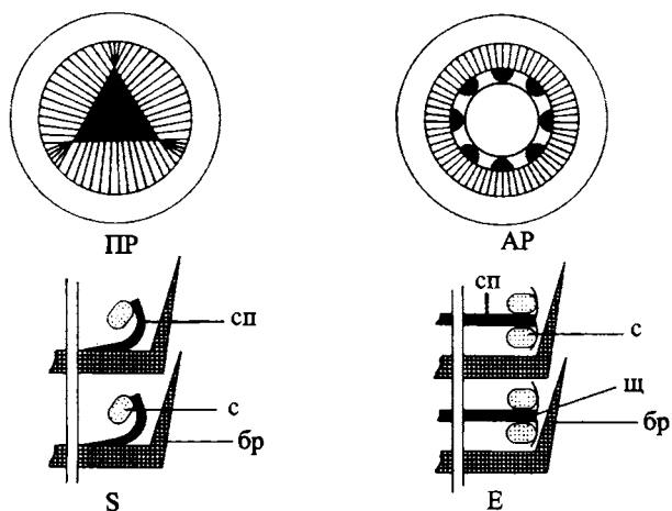
Рис. 28. Основные признаки отличия классов в отделе Equisetophyta, а также особенности строения спорофилла.
