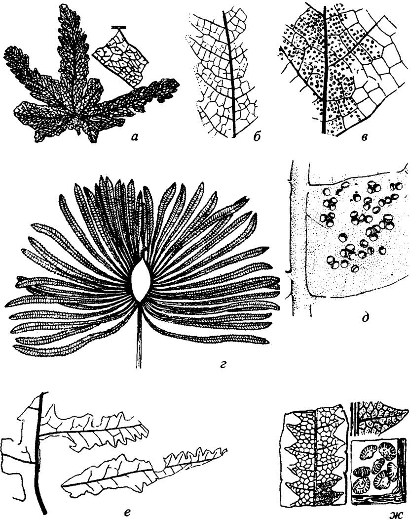
Рис. 47. Класс Polypodiopsida (P—Q). Вайи родов Clathropteris (a—v) и Dictyophyllum (z—ж):
