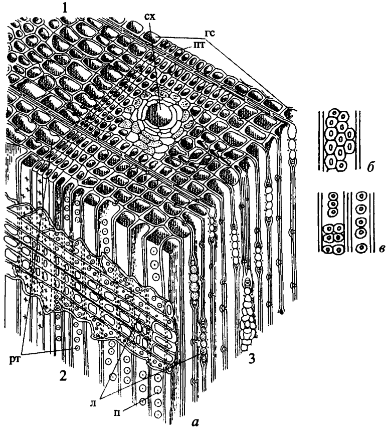
Рис. 81. Отдел Pinophyta (С—Q).
