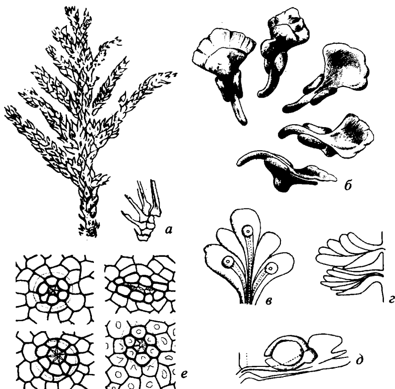
Рис. 83. Отдел Pinophyta (C—Q).
