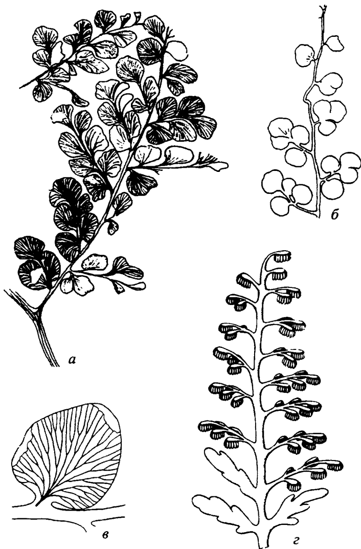
Рис. 64. Отдел Lyginopteridophyta ( D_3-K_1 ).
