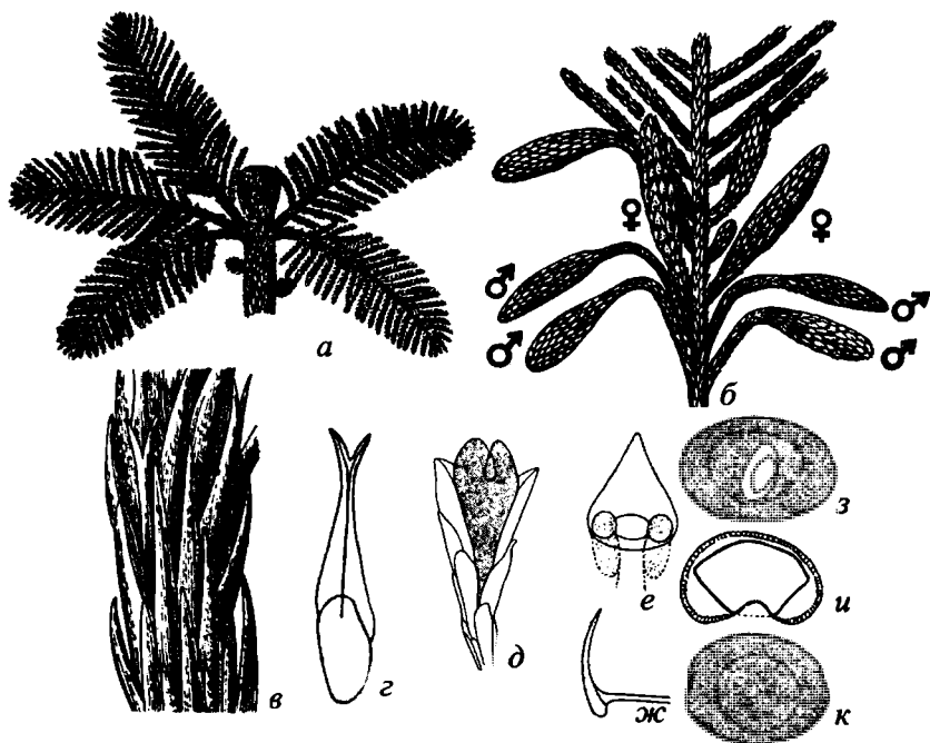
Рис. 82. Отдел Pinophyta (C—Q).
