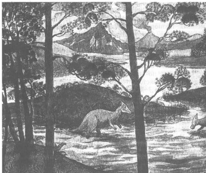
Рис. 95. Маастрихтский ландшафт Северо-Востока России (Герман, 2006)
