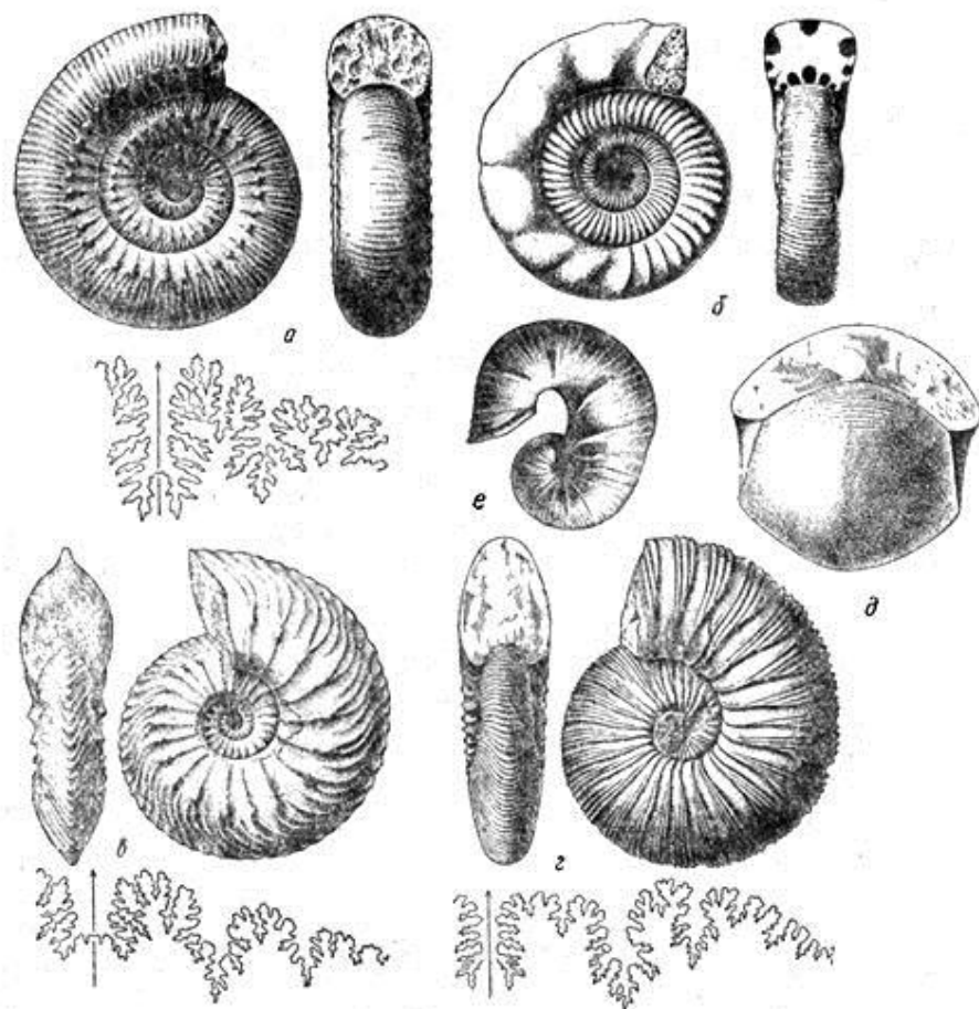
Отряд Ammonitida; а — Stephanoceras (средняя юра); б — Perisphinctes (поздняя юра); в — Cardioceras (поздняя юра); е — Virgalites (поздняя юра); д — Cadoceras (поздняя юра); е — Scaphites (мел);
