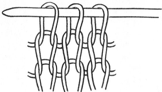
Рис. 1. Лицевая сторона вязаного полотна
