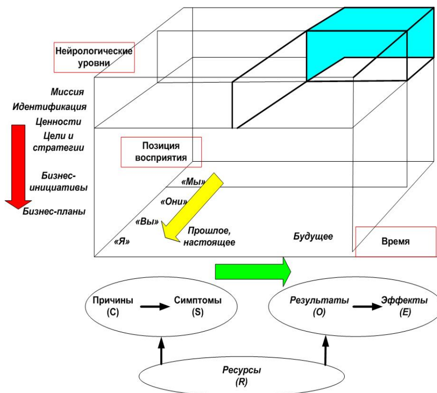
Рис. 3. Куб Гринфельда
