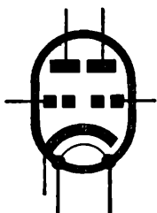
Двойной триод с общим катодом
