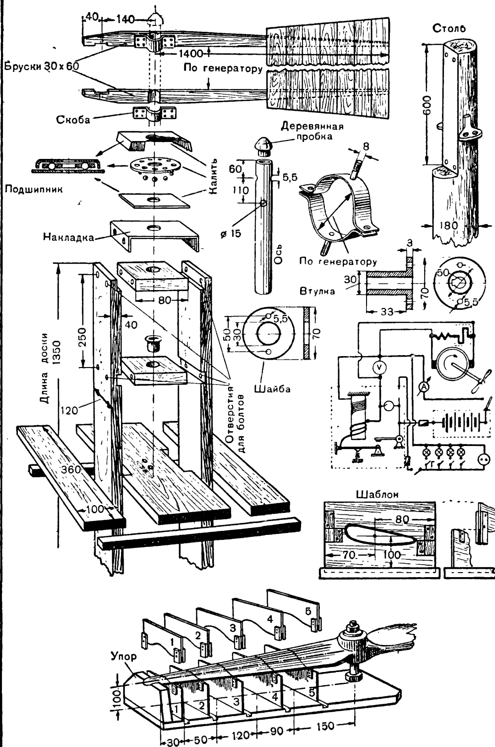
Детали ветроэлектростанции.
