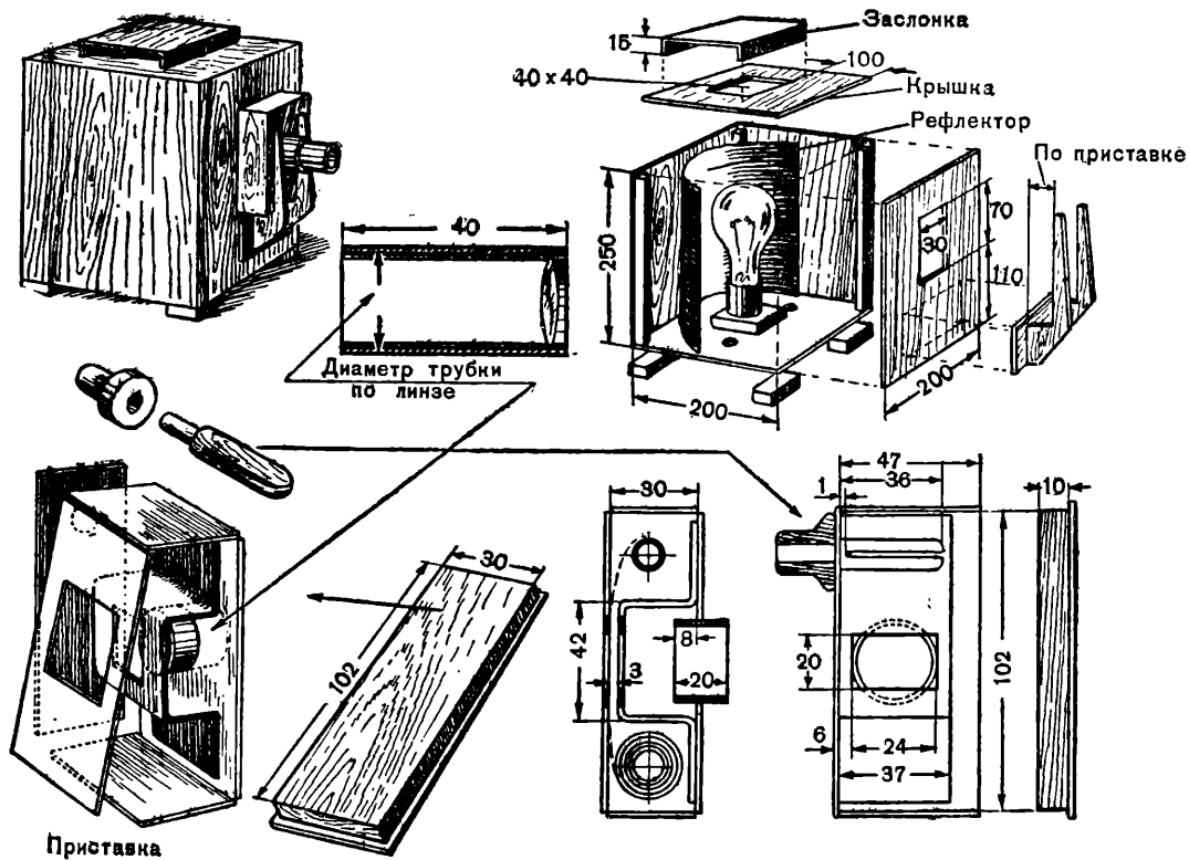
Фильмоскоп.
