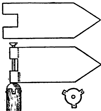
Самодельный флюгер.
