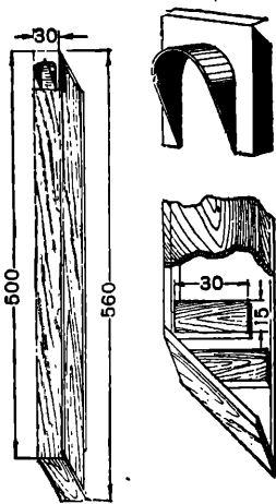
Перископ.
