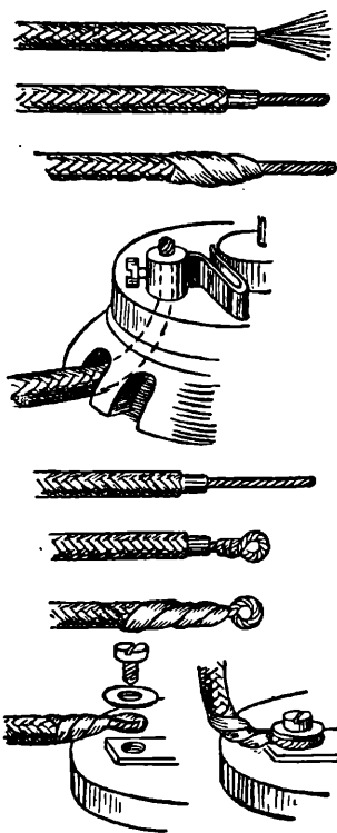
Заделка концов у провода тычком и петелькой.
