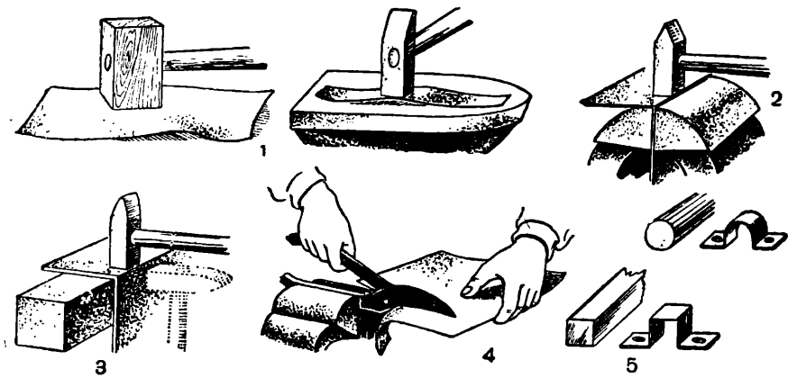
Работа с жестию: 1 — выпрямление жести; 2, 3 — сгибание под прямым углом; 4 — резание жести ножницами; 5 — изготовление скоб из жести.
