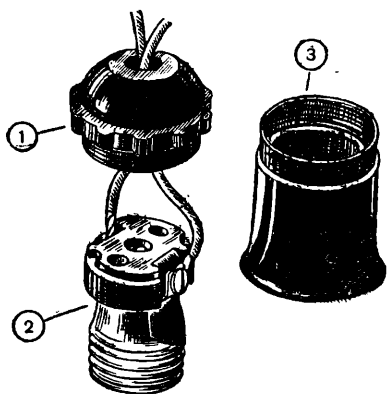
Зарядка патрона из пластмассы: 1 — крышка; 2 — патрон; 3 — чехол.
