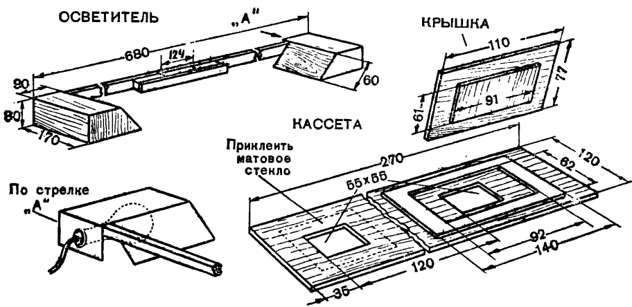
Осветитель и кассета к фотоувеличителю.
