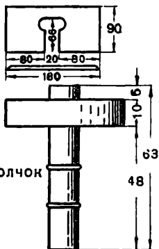
Угловая перегородка
