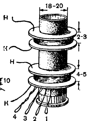
Детекторный приемник с простейшим вариометром.
