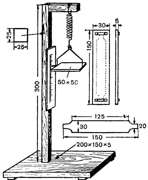
Динамометр.
