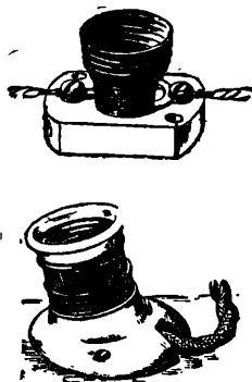
Зарядка иллюминационного и настенного патронов.
