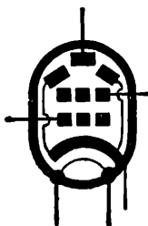
Двойной триод с общим катодом
