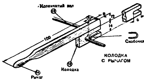
Передаточное устройство.
