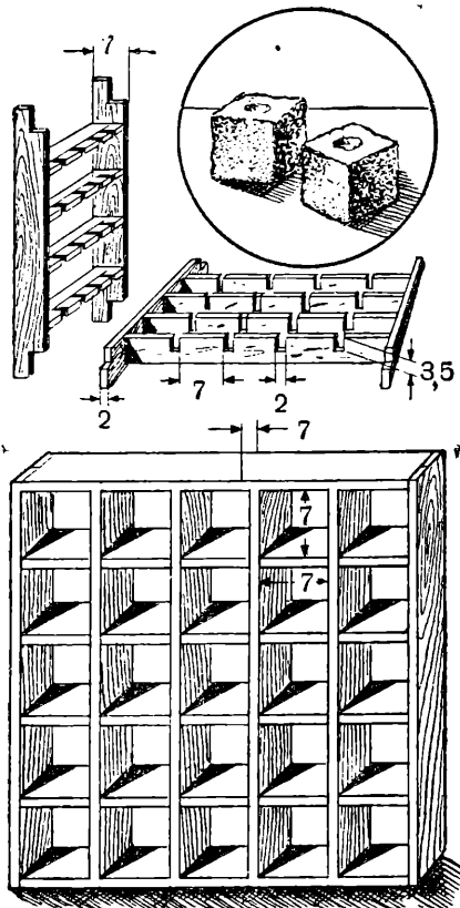
Станок для изготовления торфоперегнойных горшочков.
