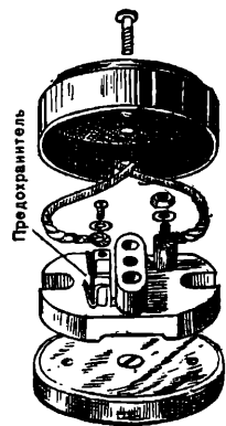
Штепсельная розетка.
