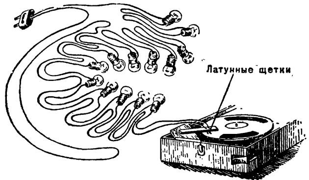
Устройство для переключения гирлянд на елке.
