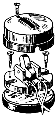
Выключатель из пластмассы с перекидным рычажком.
