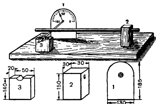
Прибор для измерения коэффициента линейного расширения.
