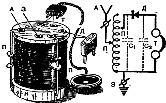
Детекторный приемник с двумя переключателями.
