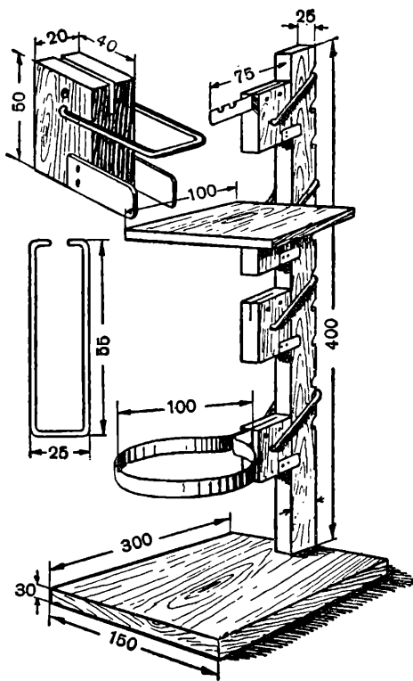
Лабораторный штатив.
