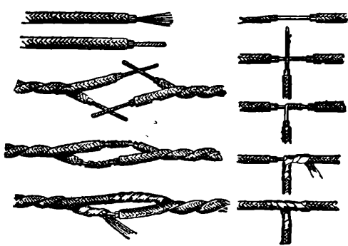
Сращивание и ответвление проводов.
