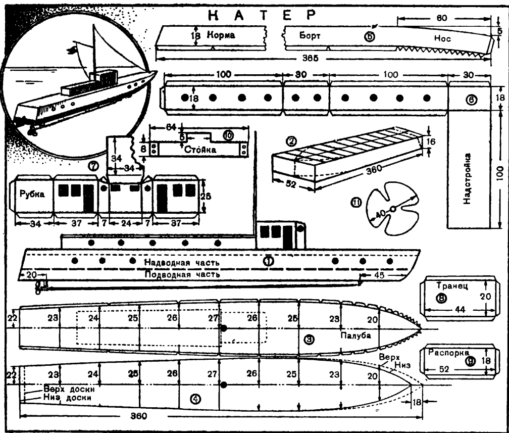
Модель катера.
