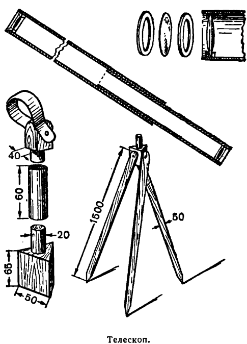
Телескоп.
