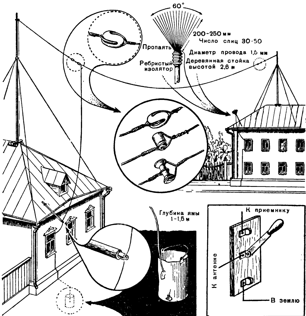
Антенны: Г-образная и метелочная; заземление; грозопереключитель.
