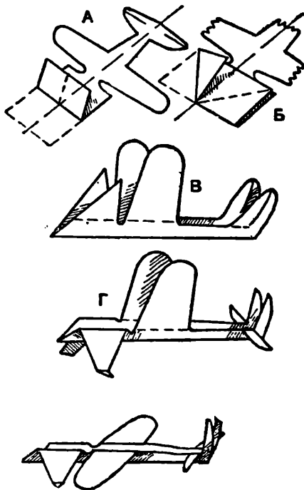
Буквами обозначена последовательность сборки простейшей модели планера.
