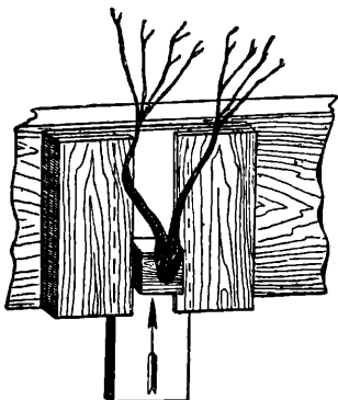
Основные типы крепления декораций. Внизу показан движок, посредством которого можно поднимать на ширму декоративную деталь на глазах у зрителя. Изготовляется из фанеры.
