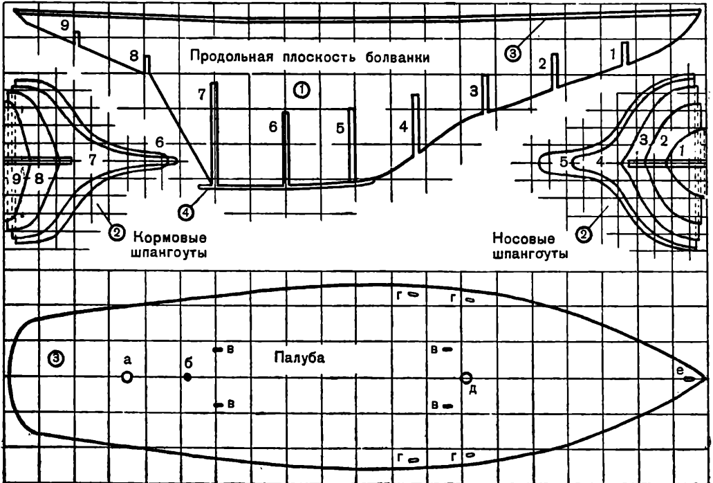
Модель яхты:
