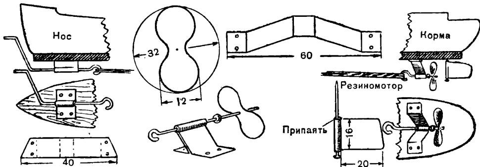
Крепление резинового мотора к контурным моделям.
