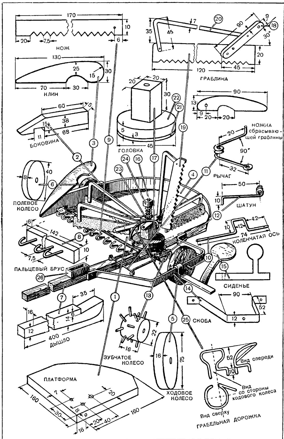
Модель жатки-самосброски.
