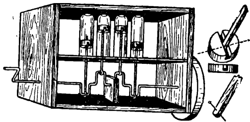
Модель четырехцилиндрового двигателя.
