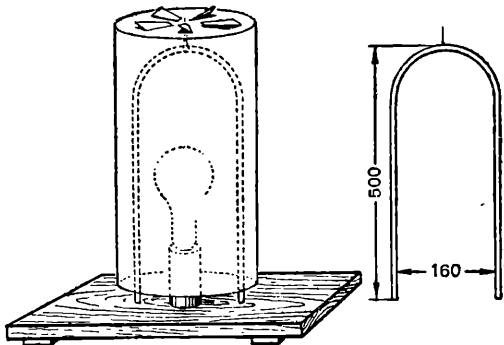
Прибор для демонстрации конвекции.
