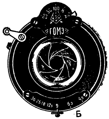
Диафрагма: А — отверстие диафрагмы полностью открыто; Б — отверстие уменьшено.
