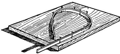
Приспособление для изгибания рейки.
