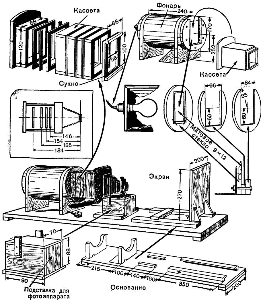
Фотоувеличитель с аппаратами „Москва-1“ и „Москва-2“.
