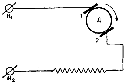
Схема соединения обмоток электромоторчика.
