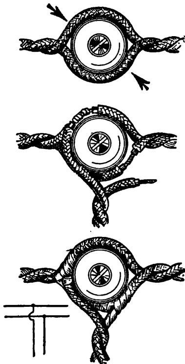
Параллельное ответвление проводов.
