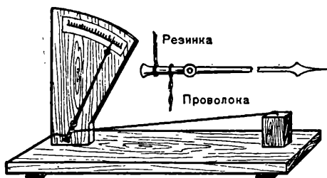
Пирометр.
