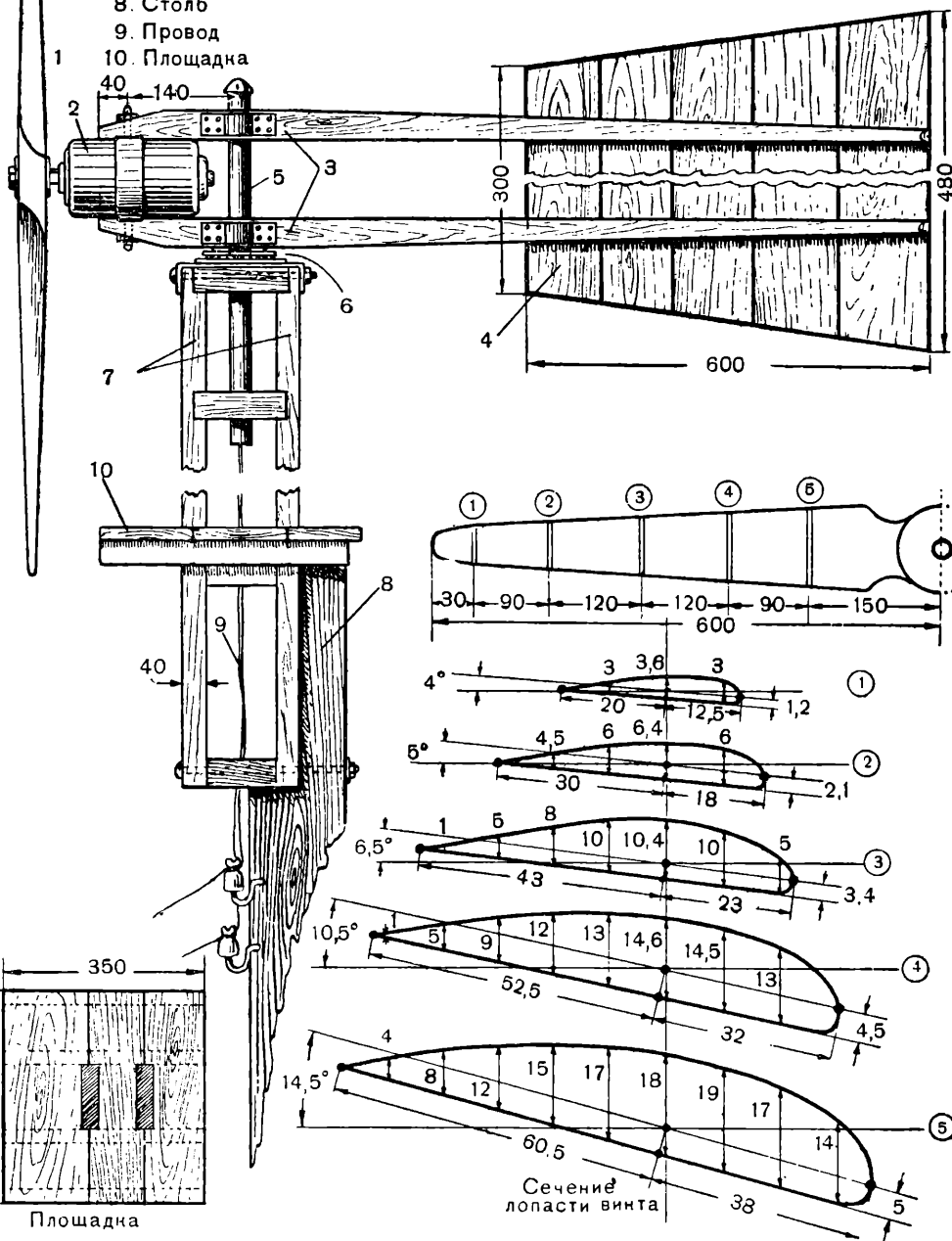
Ветроэлектростанция.
