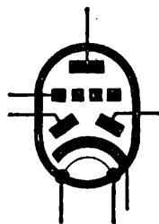
Двойной диод-триод
