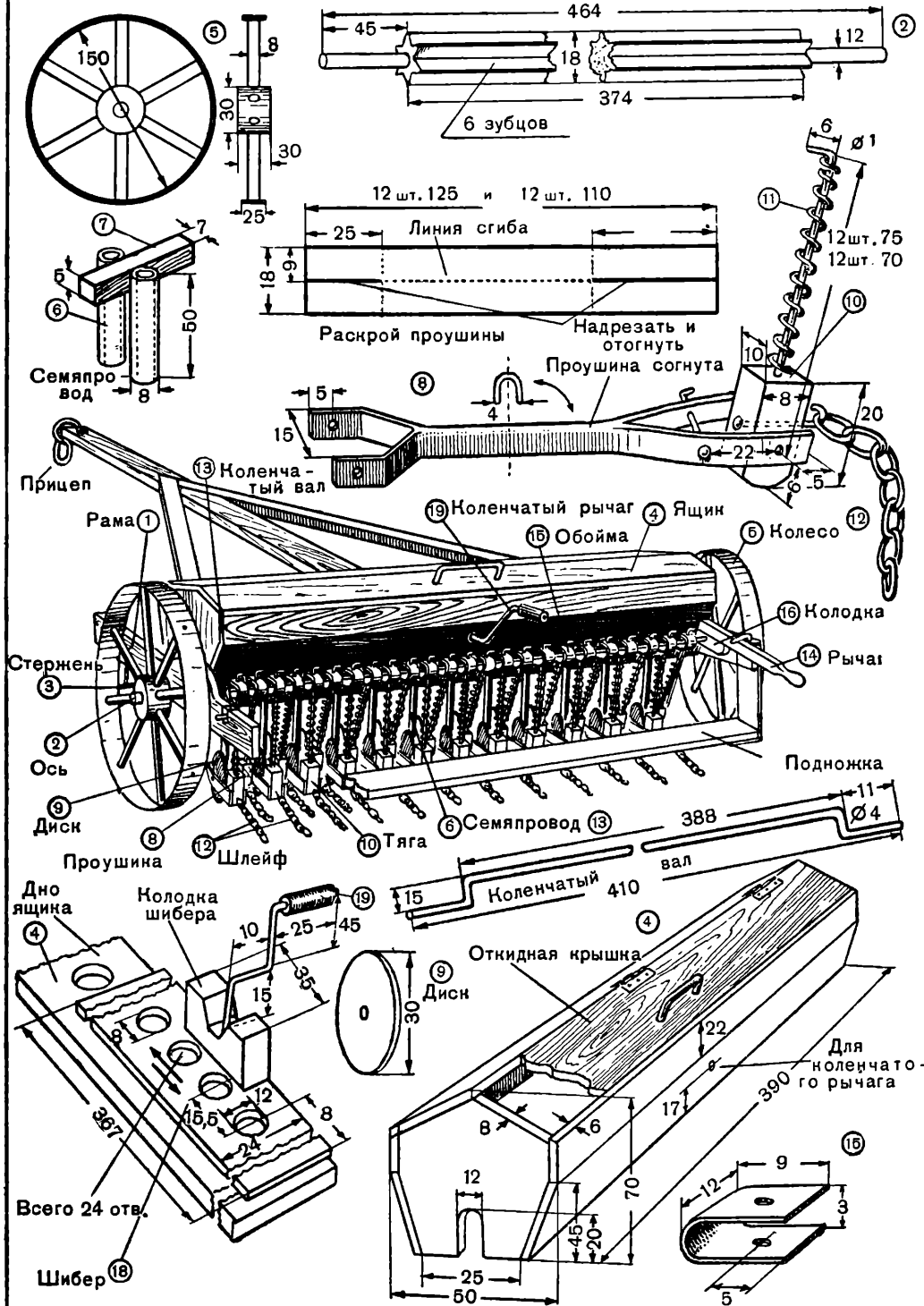
Модель тракторной 24-рядной сеялки.
