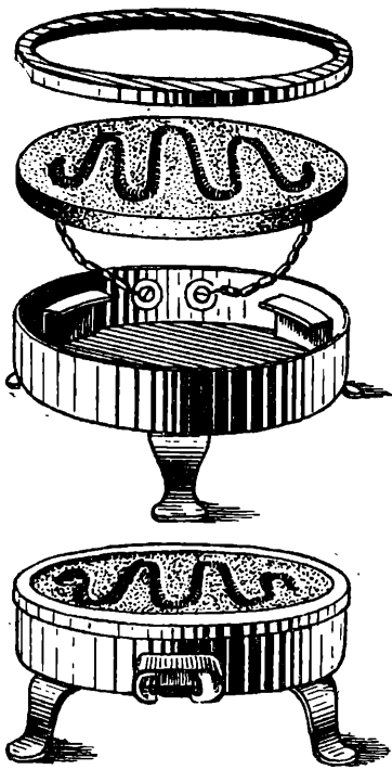
Электрическая плитка.
