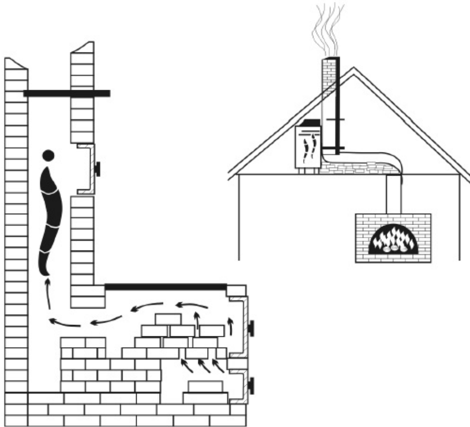
Коптильня в дымоходной трубе
