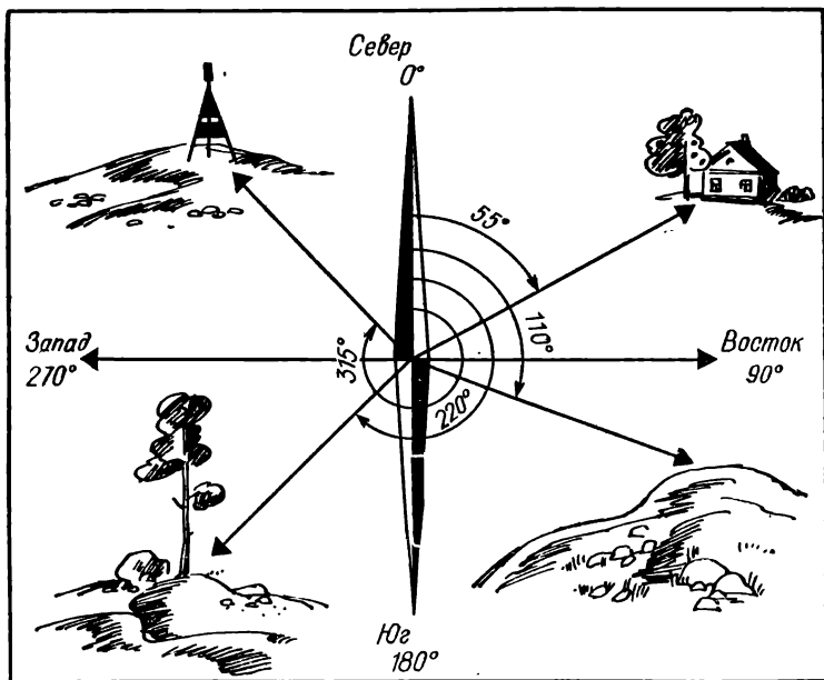
Рис. 20. Магнитные азимуты
