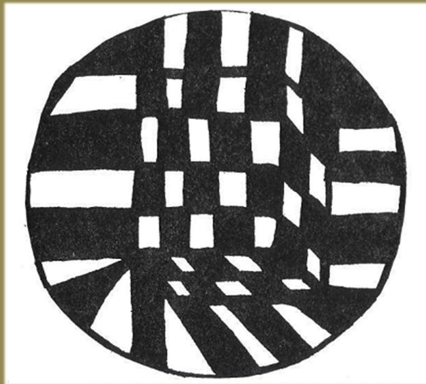
Диаграмма 4: Четырехмерный куб, используемый приверженцами культа Черного Змея
