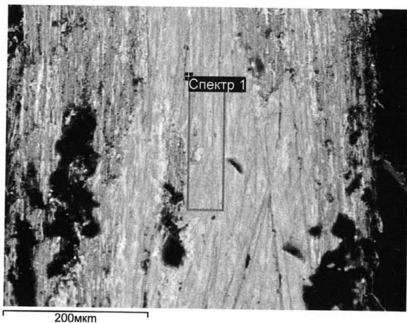
Рис 3. Увеличенное изображение среза монеты (акче Мухаммеда Гирея I. 922 г.х. Группа А)
