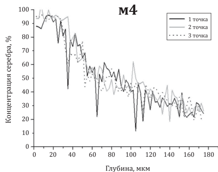
Рисунок 9. Зависимость концентрации серебра от глубины измерения для образца м4 – пражского гроша Вацлава IV (в трёх точках)
