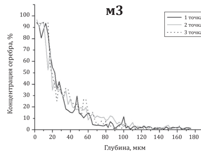
Рисунок 8. Зависимость концентрации серебра от глубины измерения для образца м3 – львовского полугроша Ягайло (в трёх точках)
