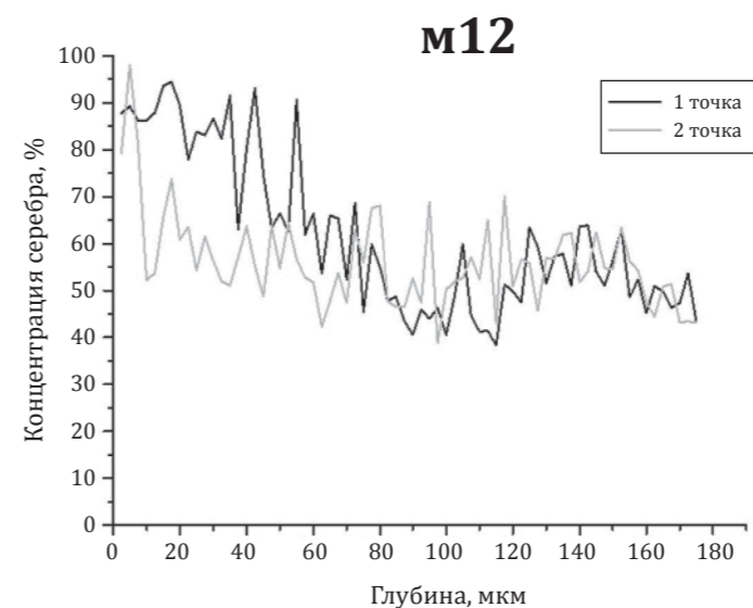
Рисунок 18. Зависимость концентрации серебра от глубины измерения для образца м12 – неопределённого крымского данга (в двух точках)
