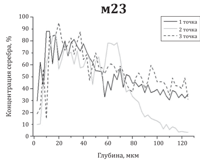
Рисунок 29. Зависимость концентрации серебра от глубины измерения для образца м23 – пенязя Владимира Ольгердовича начала 1390-х (в трёх точках)
