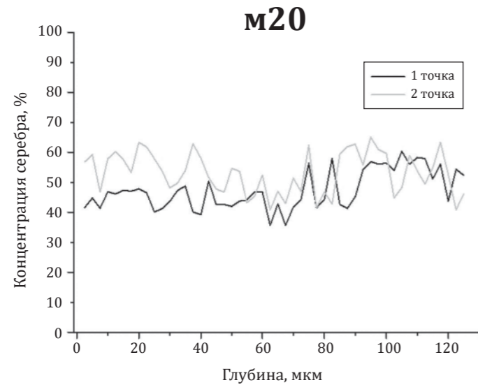
Рисунок 21. Зависимость концентрации серебра от глубины измерения для образца м20 – данга Дервиша чекана Хаджи-Тархана (в двух точках)
