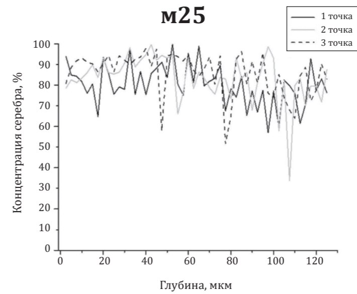
Рисунок 31. Зависимость концентрации серебра от глубины измерения для образца м25 – неизвестной денги нижегородского круга начала XV века (в трёх точках)
