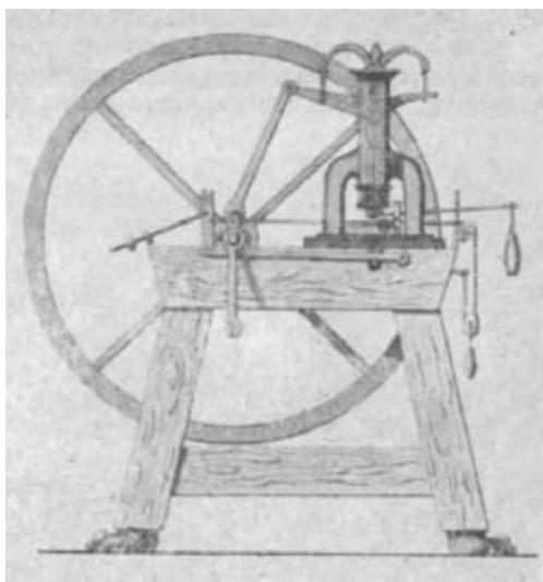
Рис. 165. Монетный кривошипный пресс И. А. Неведомского 1811 г.
