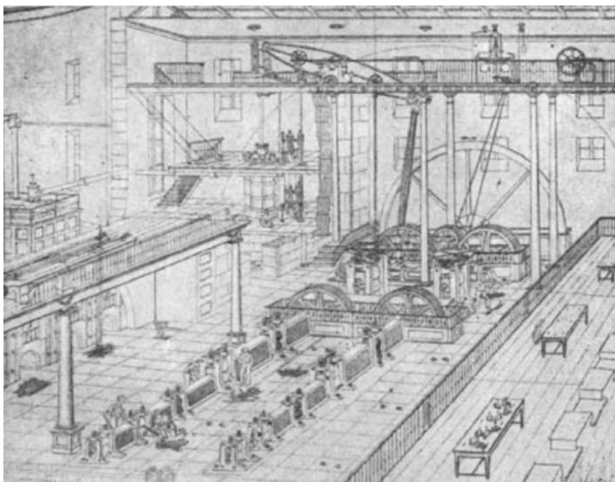
Рис. 167. Внутренний вид (разрез) здания Петербургского монетного двора в 20-х гг. XIX в. Внутри угловой башни (против собора) находилась котельная.
