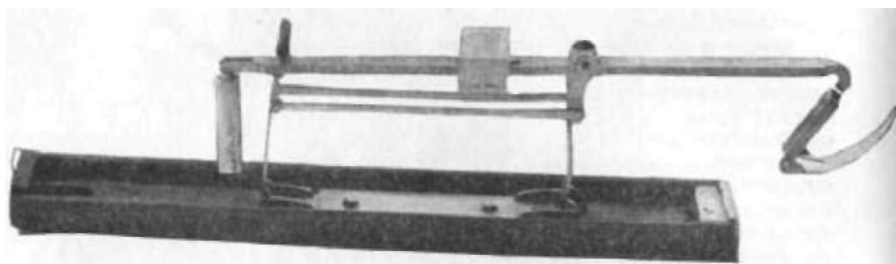
Рис. 22. Монетные весы первой половины XIX в. Франция.
