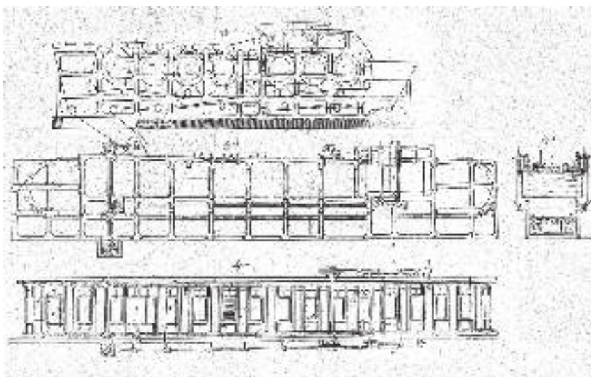
Рис. 2. Чертеж (план, разрезы) черпальной машины из спецификации патента Ш. Дено. [1879 г.]. (ЦГИА СПб. Ф. 1458. Оп. 2. Д. 576. Л. 91)
